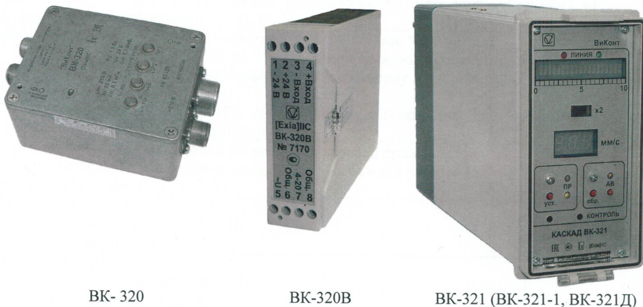
Рисунок 2 - Общий вид вторичных блоков измерения вибрации ВК-320, ВК-320В, ВК-321 (ВК-321-1, ВК-321Д)
