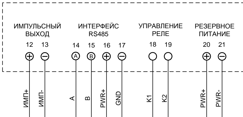
Рисунок Б.9 – Схема подключения интерфейсов и вспомогательных цепей «Меркурий 204»
