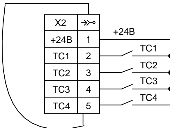
Рисунок Б.13 – Схема подключения дискретных входов «Меркурий 204», «Меркурий 234» с функциями телемеханики
