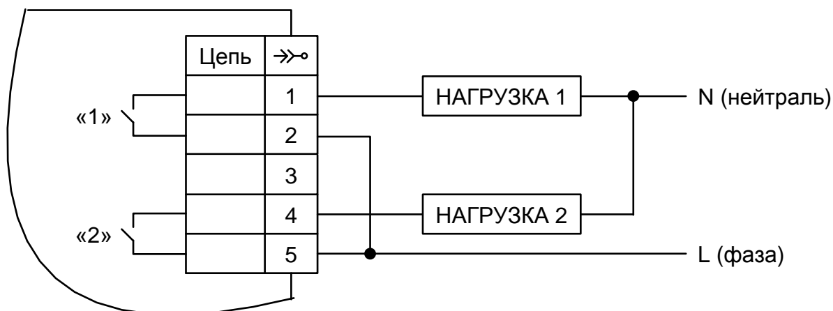
Рисунок Б.14 – Схема подключения дискретных выходов «Меркурий 204», «Меркурий 234» с функциями телемеханики
