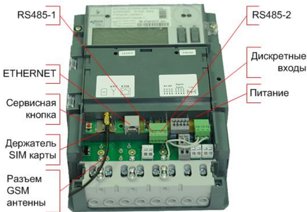
Рисунок 4.2 Вид счетчика с функциями телемеханики с элементами подключения
