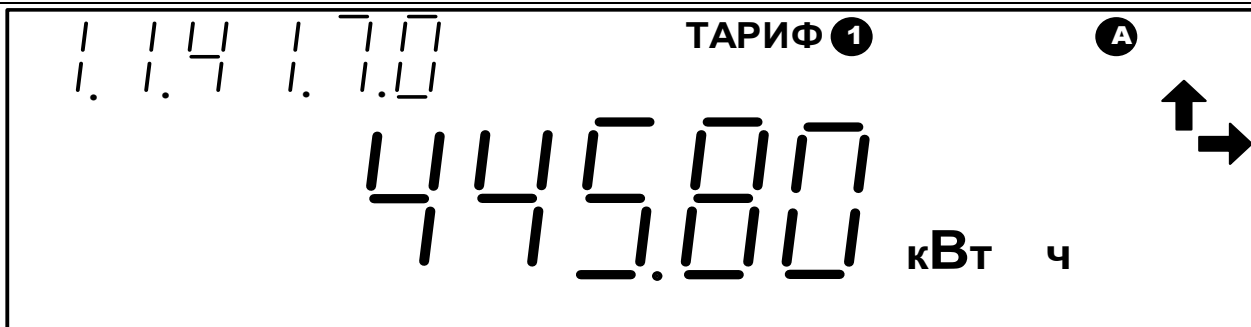
Рисунок 4.5 – Отображение накопленной энергии
