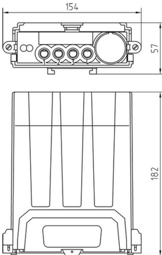
Рисунок А.2 – Габаритный чертеж счетчика «Меркурий 208»
