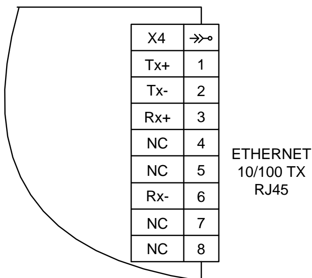
Рисунок Б.12 – Схема подключения интерфейса Ethernet «Меркурий 204», «Меркурий 234» с функциями телемеханики
