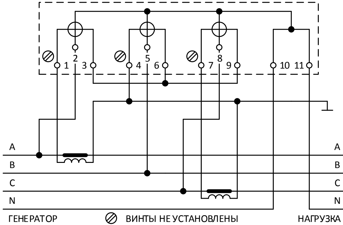
Рисунок Б.5 – Схема подключения счетчиков «Меркурий 234», включение через два трансформатора тока
