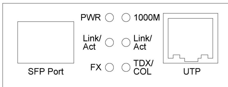
Рисунок 1. Фронтальная панель.
