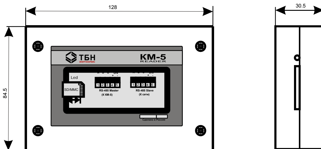
Рисунок 1.1 — Внешний вид и габаритные размеры адаптера
