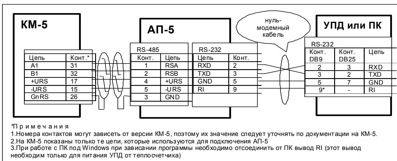
Рисунок Б.1— Схема монтажа адаптера периферии АП-5
