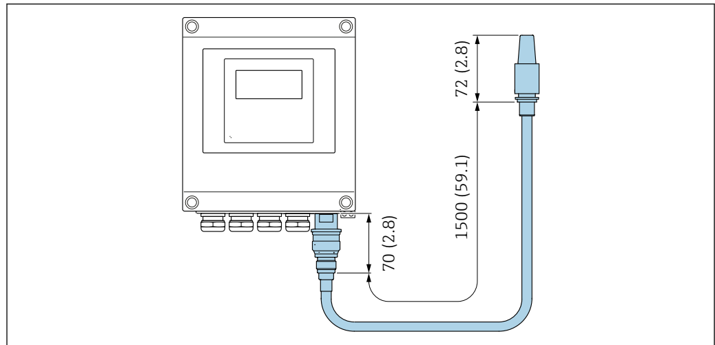
30 Единица измерения, мм (дюйм)
