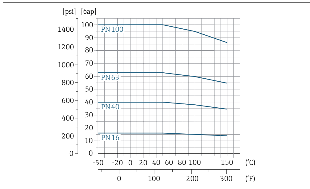
22 С материалом фланца 1.4404 (316, 316L)
