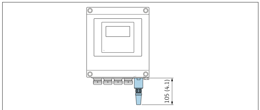
29 Единица измерения, мм (дюйм)
