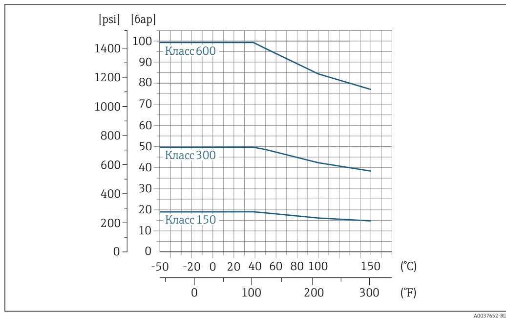
23 С материалом фланца 1.4404 (316, 316L)
