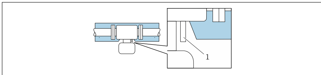
24 Теплоизоляция с открытой удлинительной шейкой и измерительной ячейкой для давления
