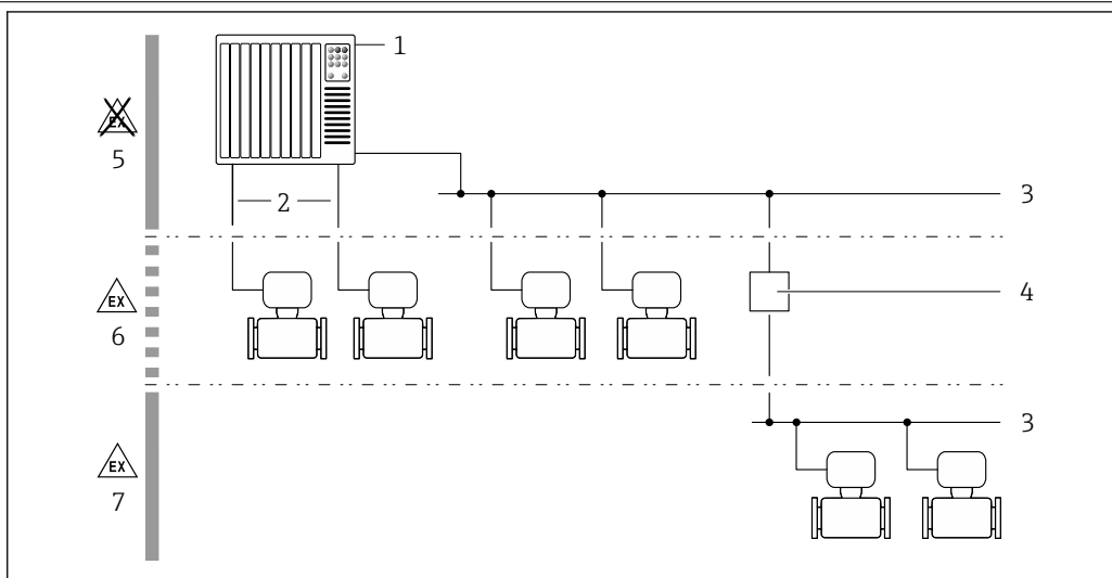
2 Возможности интегрирования измерительных приборов в систему
