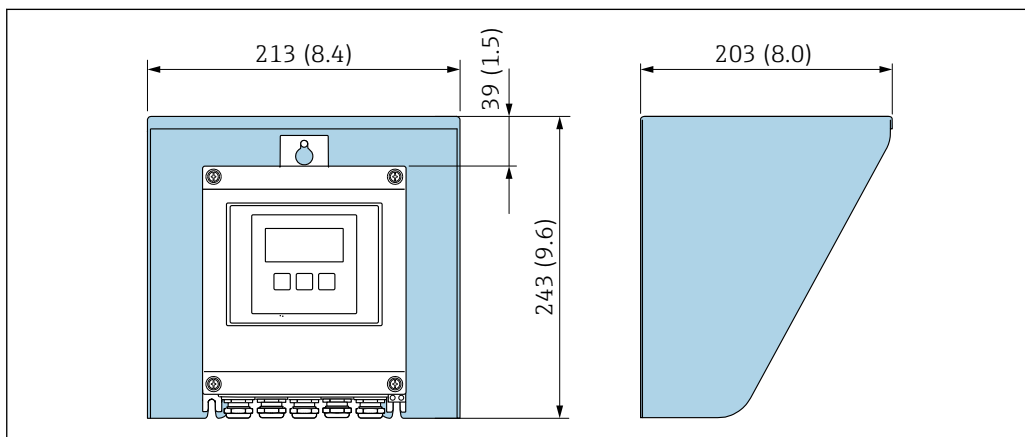
21 Защитный козырек от атмосферных явлений для Proline 500 в цифровом исполнении
