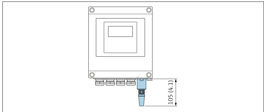
▣ 26 Единица измерения, мм (дюйм)
