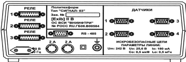
Рис.2. Вид задней панели блока информационного
