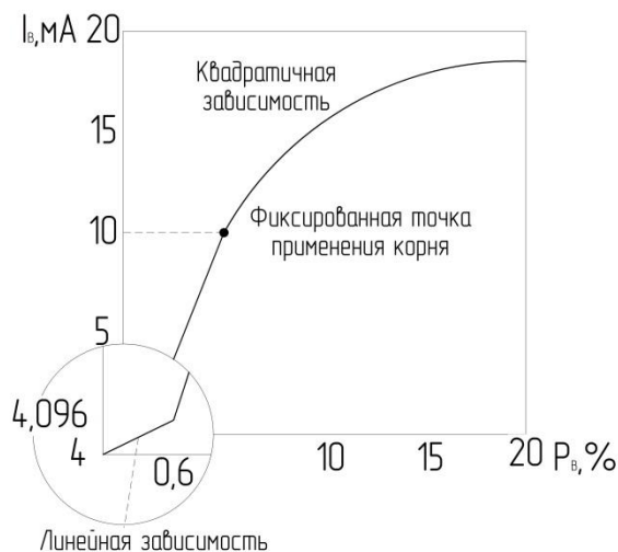
Рисунок 37 – График «КВЛИ2»
