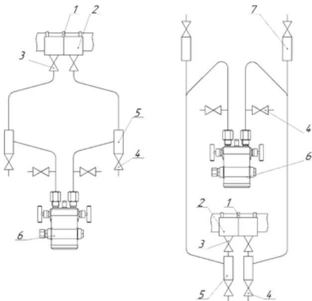
Рисунок 8 – Схема соединительных линий при измерении газа
