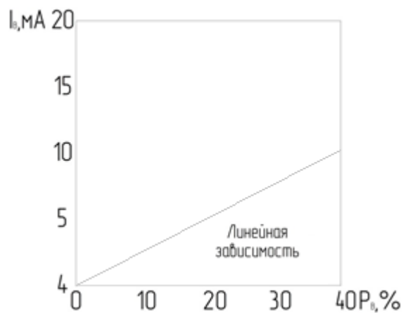
Рисунок 31 – График «ЛИН»
