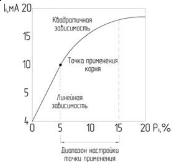
Рисунок 33 – График «КВЛИН»
