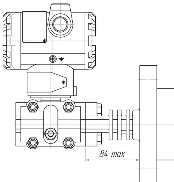
Рисунок Д.5 – Габаритные и присоединительные размеры специального фланцевого исполнения датчиков давления ЭМИС-БАР 163. Размеры фланца указаны на страницах 108 – 111.
