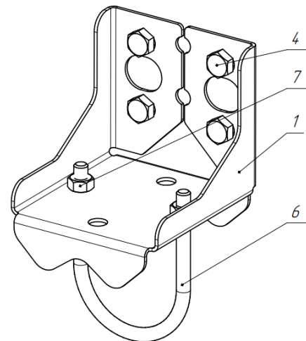
Рисунок Е.4 – Кронштейн угловой в комплекте с КМЧ
