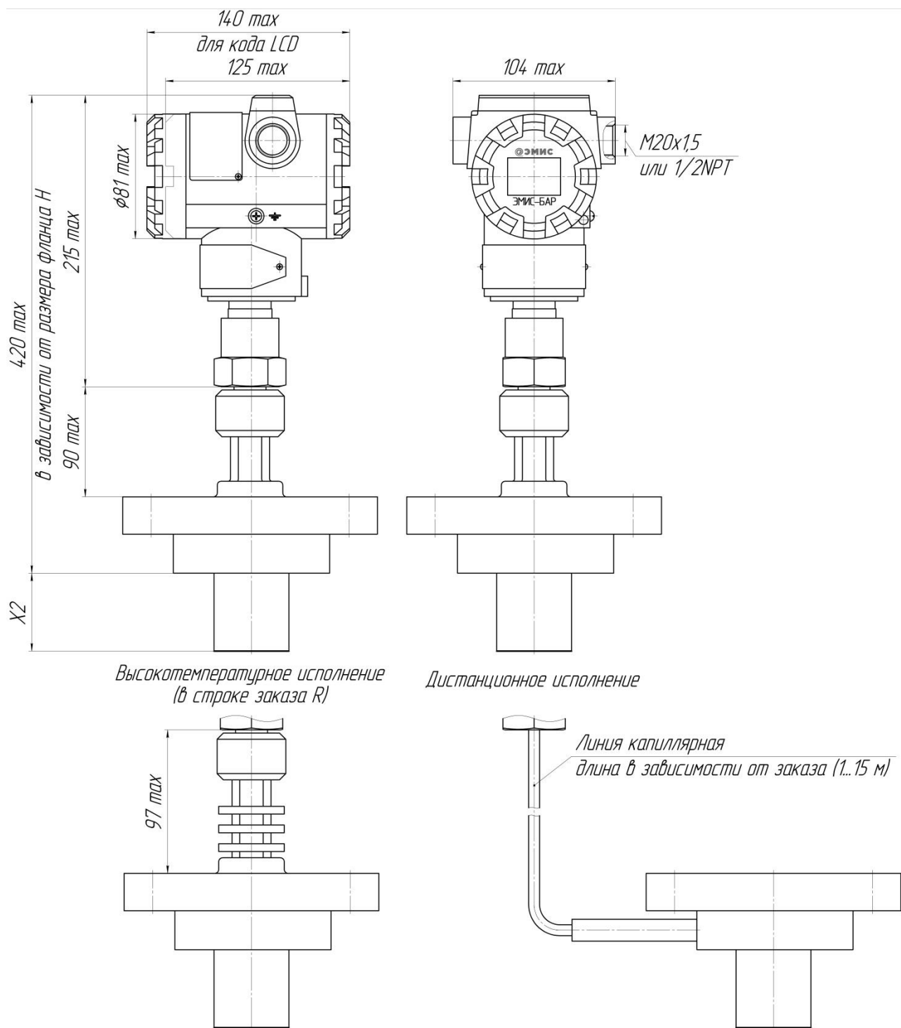
Рисунок Д.8 – Габаритные и присоединительные размеры специального фланцевого исполнения датчиков давления ЭМИС-БАР 174 и 176. Размеры фланца указаны на страницах 108 – 111.
