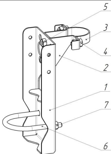
Рисунок Е.1 – Кронштейн горизонтальный в комплекте с КМЧ
