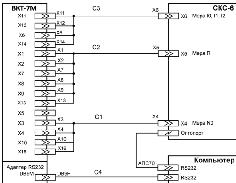
Рисунок 8.1 – Схема поверки
