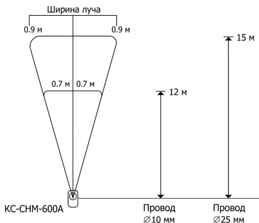
Рис. 1 – Зона измерения
