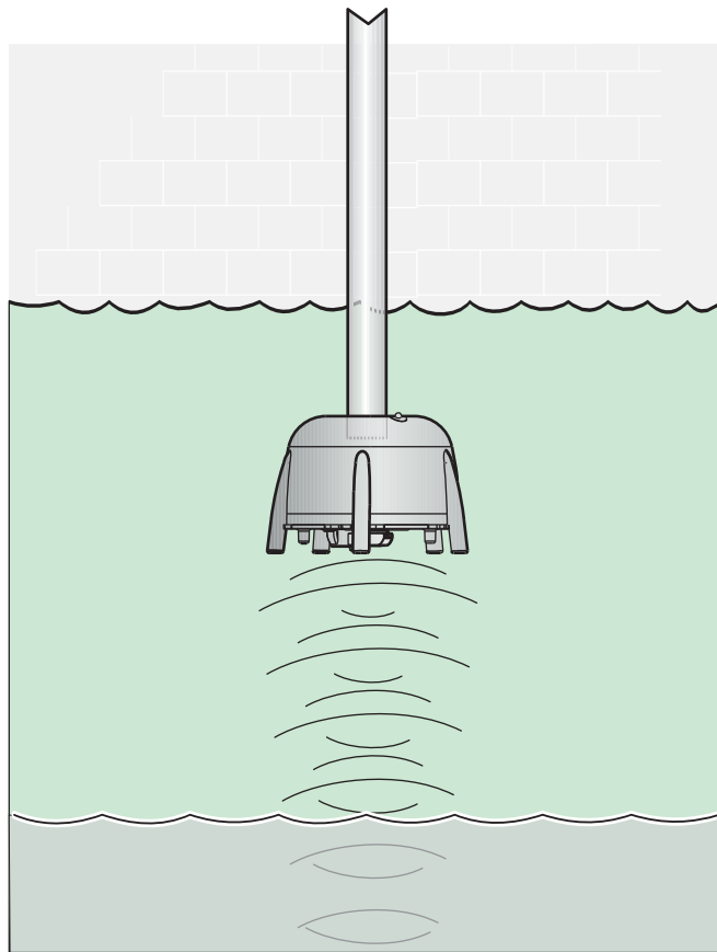
Рисунок 2 Принцип работы
