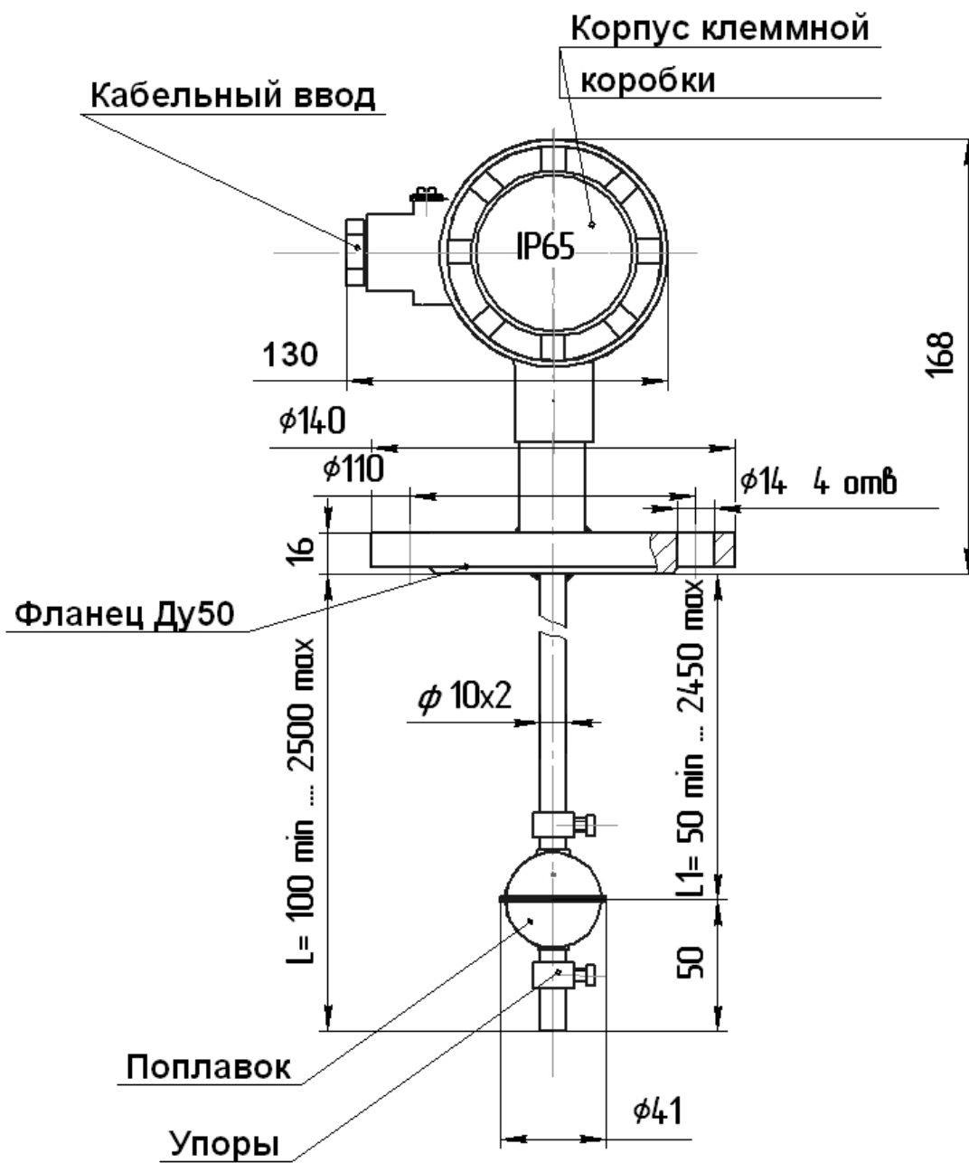
Рисунок А.1 - СУЖ-П-С с одним поплавком
