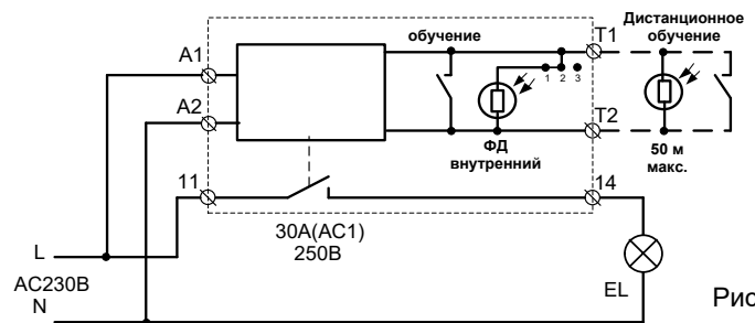
Схема подключения
