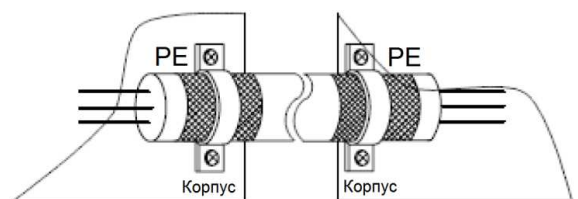
Рисунок 19 – Способ крепления кабеля
