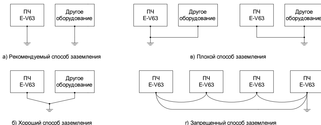
Рисунок 9 – Способы заземления
