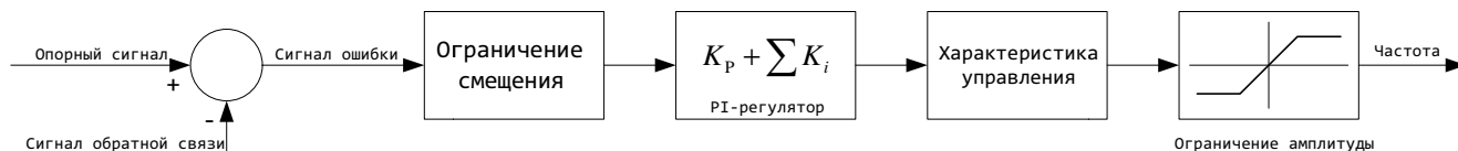
Рисунок 74 – Структура ПИ-регулятора
