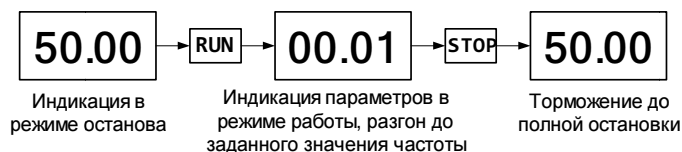
Рисунок 50 – Алгоритм запуска/остановки ПЧ
