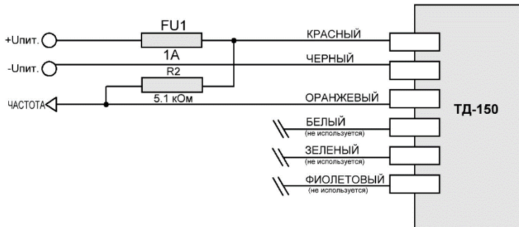
ПРИЛОЖЕНИЕ 4. Схема подключения измерителя в частотном режиме с “подтяжкой” через резистор
