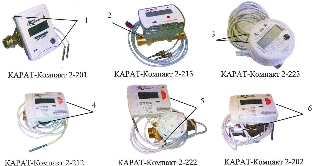
1 – 6 Места пломбирования при выпуске из производства
