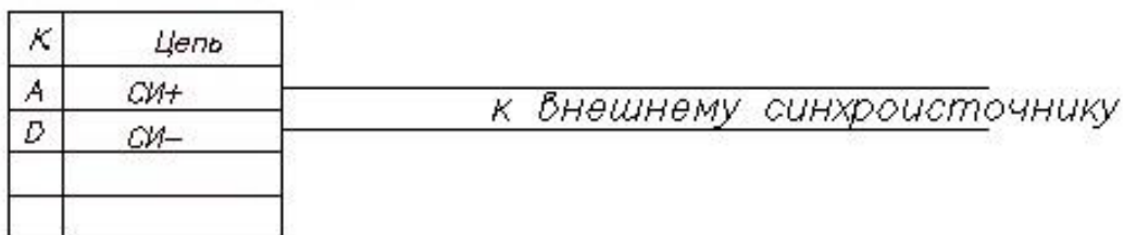
Схема кабеля синхронизации ИУСЕ 685621.052 (-02)
