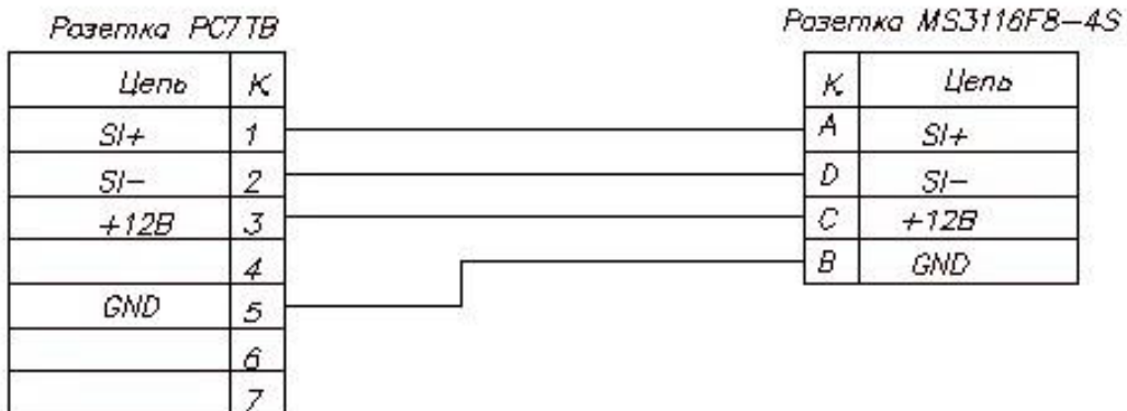
Схема кабеля Лакколит ИУСЕ 685621.051
