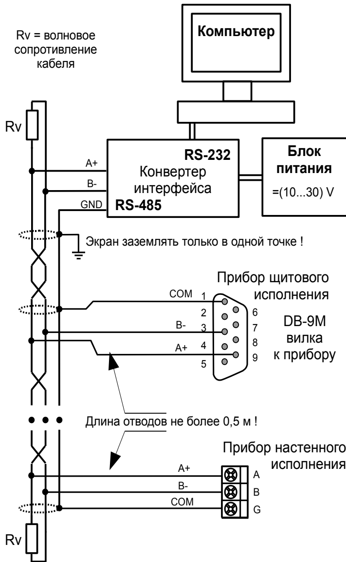
Рисунок С.7 - Включение приборов с интерфейсом RS-485 в локальную сеть
