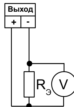
Рисунок I.3 - Схема подключения при проверке аналогового выхода
