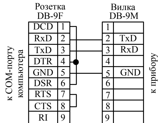
Рисунок С.9 - Кабель для подключения прибора щитового исполнения с интерфейсом RS-232 к COM-порту компьютера
