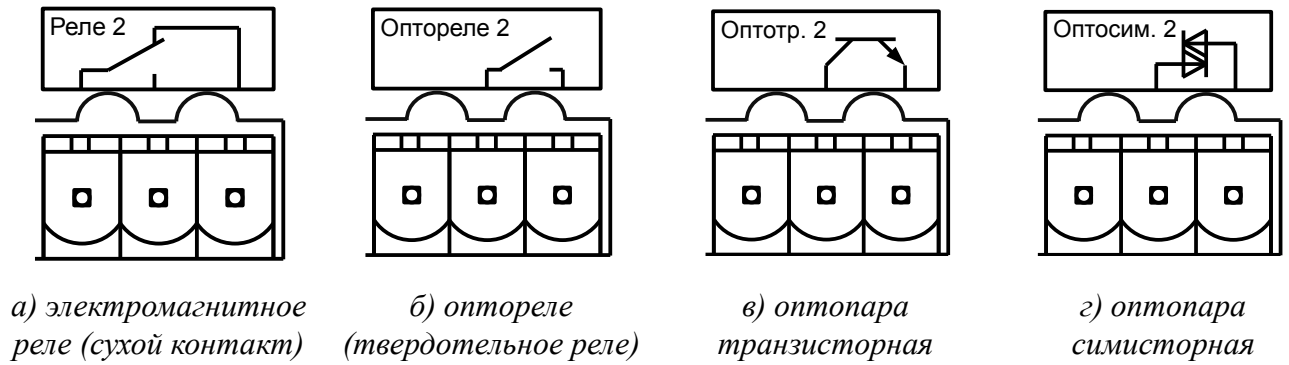
Рисунок С.4 - Маркировка дискретных выходов прибора щитового исполнения
