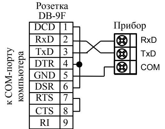
Рисунок С.8 - Включение приборов настенного исполнения с интерфейсом RS-232 к COM-порту компьютера
