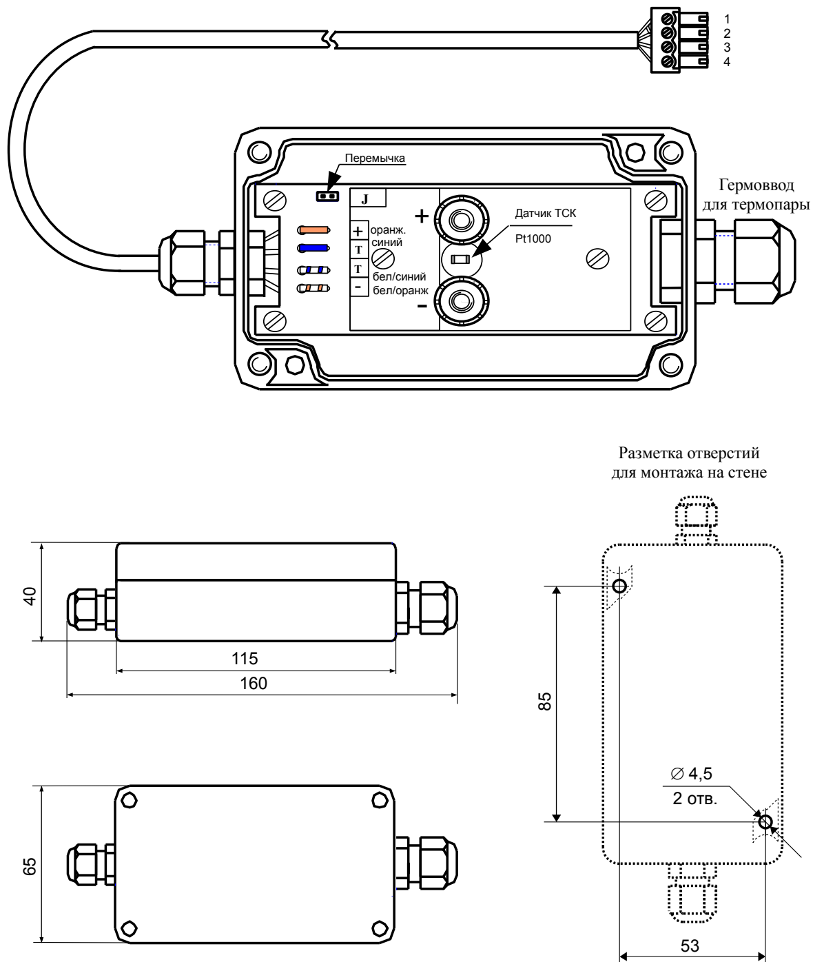
Рисунок D.1 - Компенсационная коробка КСК-1.4.3
