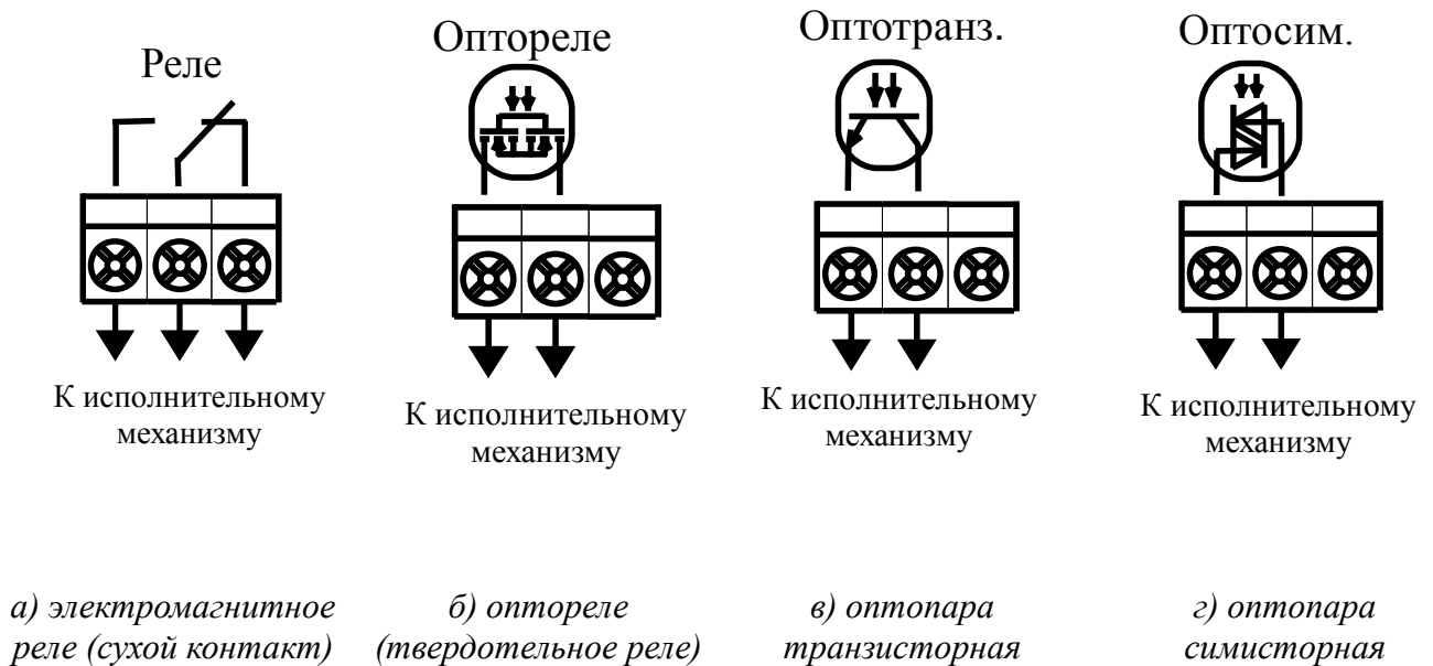
Рисунок С.5 - Маркировка дискретных выходов прибора настенного исполнения
