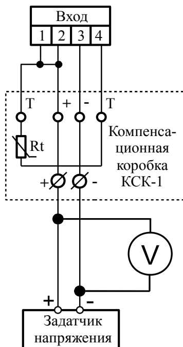
Рисунок I.2 - Схема подключения при проверке входа для сигналов от термопар
