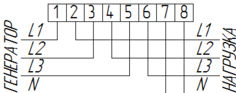
Рисунок Б.1 - Схема подключения счетчика в исполнении С
