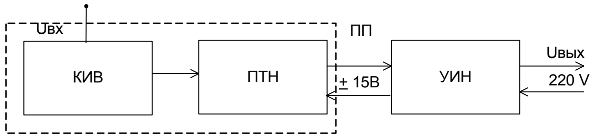
Рисунок 2.1 - Структурная схема ПВЕ.
