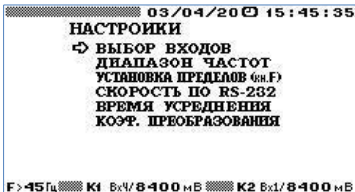
Рисунок 3.3 - Меню "Настройки"
