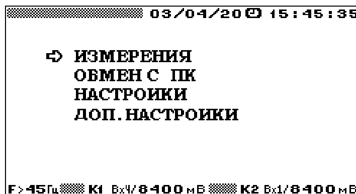
Рисунок 3.2 - Главное меню
