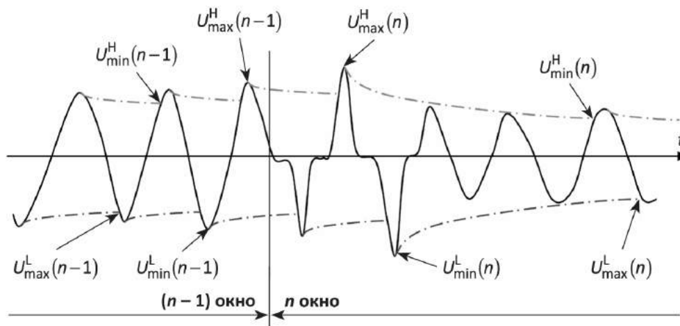
Рис. 4.8.6 Диаграмма работы прибора в режиме «АМПЛИТУДНЫЙ ДЕТЕКТОР»
