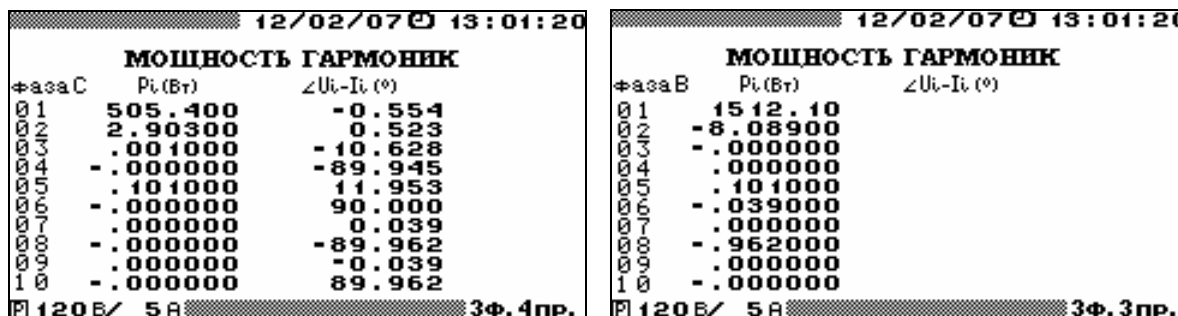
Рисунок 4.3.8 Режим отображения гармонических составляющих активной мощности для различных схем включения
