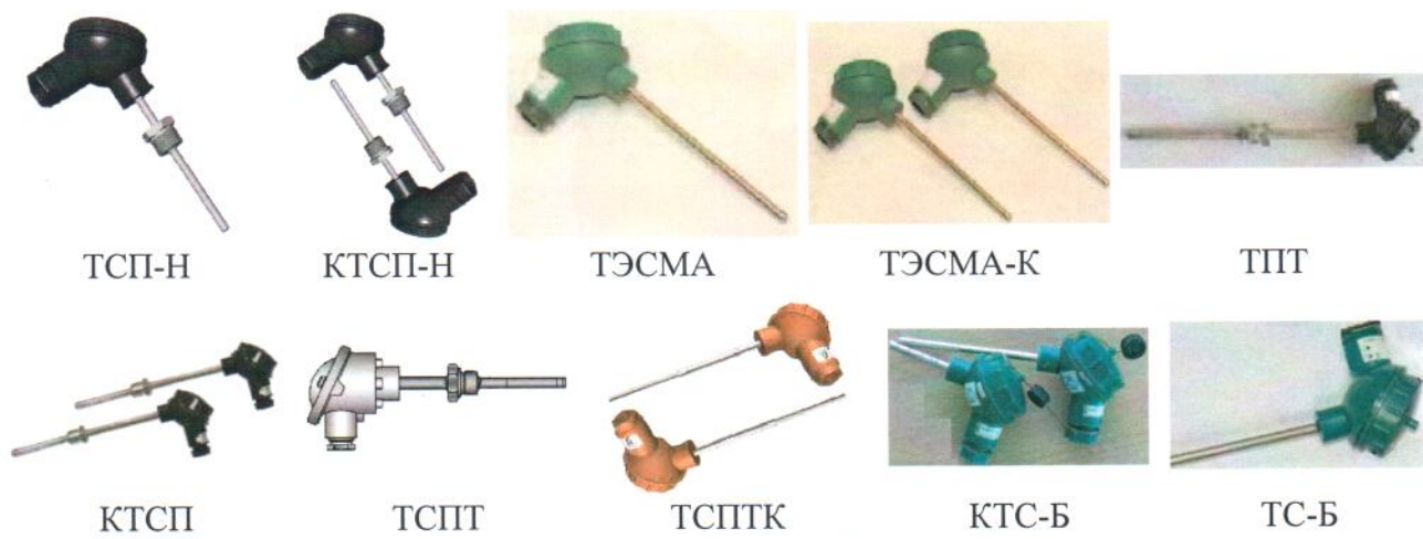
Рисунок 3 - Общий вид ТС
