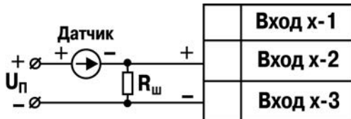
Рисунок Б.11 – Схема подключения активного датчика с токовым выходом 0...5 мА или 0(4)...20 мА
