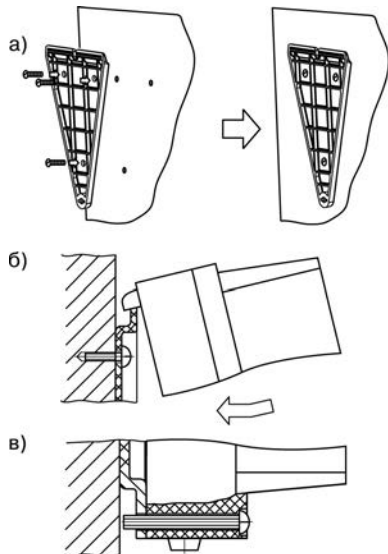
Рисунок 5.1 – Монтаж прибора настенного исполнения
