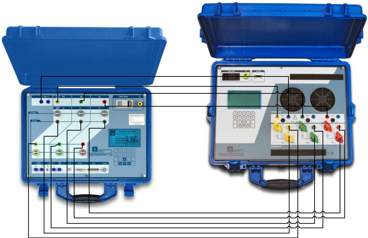
Рисунок А.2 - Схема соединения генератора «Энергоформа-3.3-120М» и прибора «Энергомонитор-3.1КМ» при токе до 12 А.
