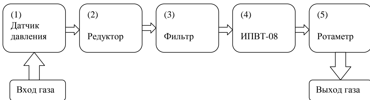
Рисунок 3.3(а) Структурная схема системы пробоподготовки газов СПГ-Н
