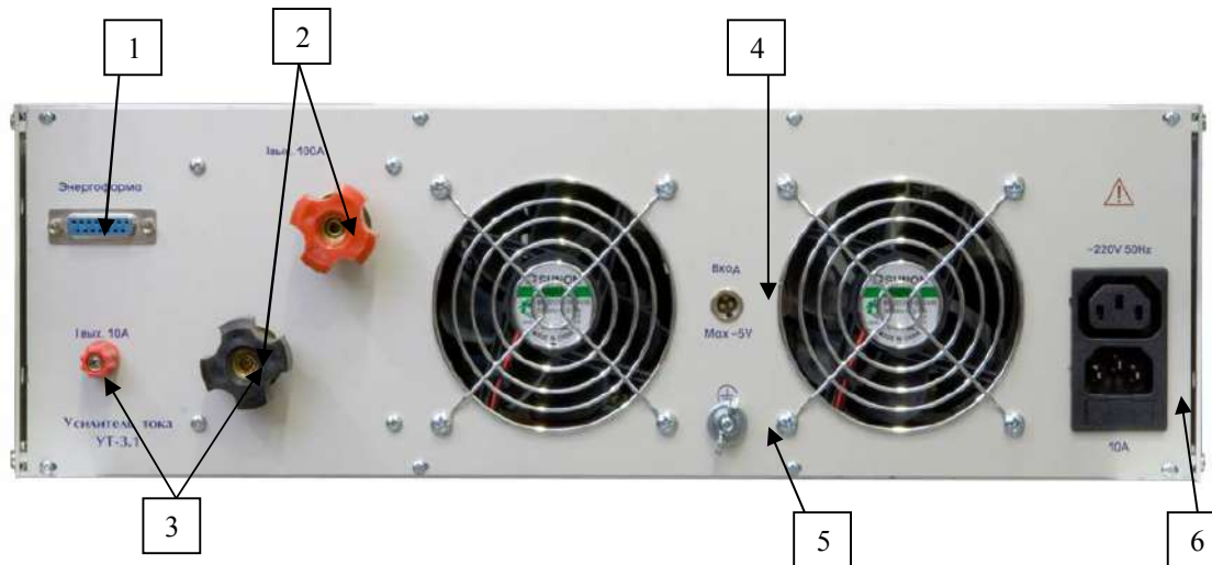
Рисунок 2.10 - Вид задней панели усилителя тока «УТ-3.1»
