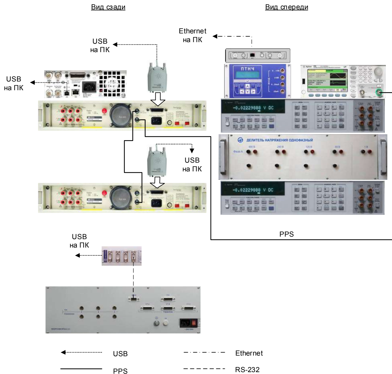
Рисунок А.6 - Схема цепей синхронизации и связи
