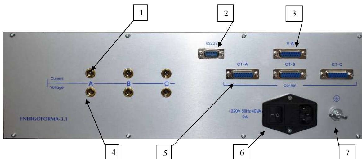
1 — соединители для передачи форм сигналов тока на усилители; 2 — соединитель интерфейса RS-232; 3 — соединитель шины управления усилителями напряжения; 4 — соединители для передачи форм сигналов напряжения на усилители; 5 — соединители шин управления усилителями тока; 6 — соединитель и тумблер питания, держатели предохранителей; 7 — соединитель заземления
