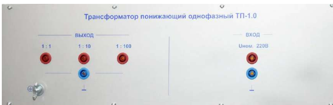
Рисунок 2.5а - Вид задней панели ТП-1.0.
