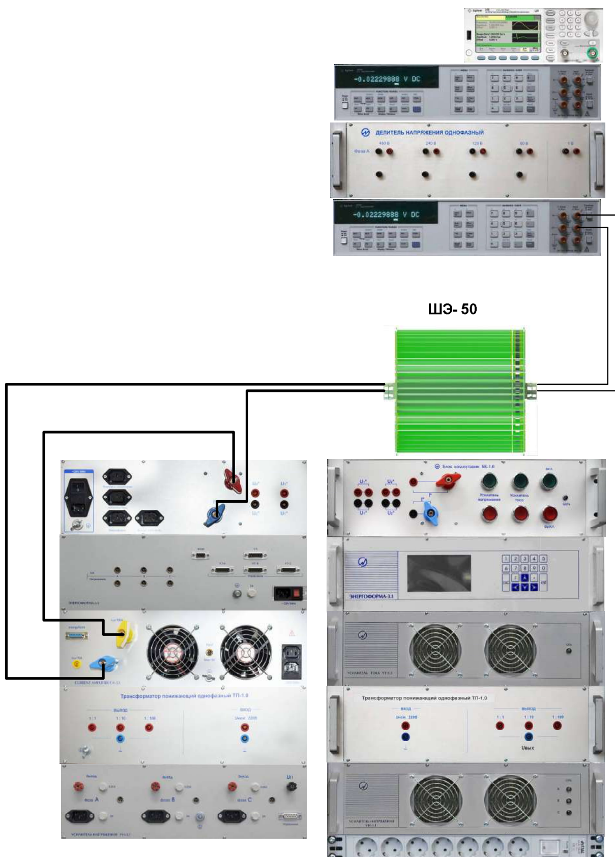
Рисунок А.2 - Схема измерительной цепи тока 50 А (перемычка на передних клеммах тока БК-1.0 не установлена!)
