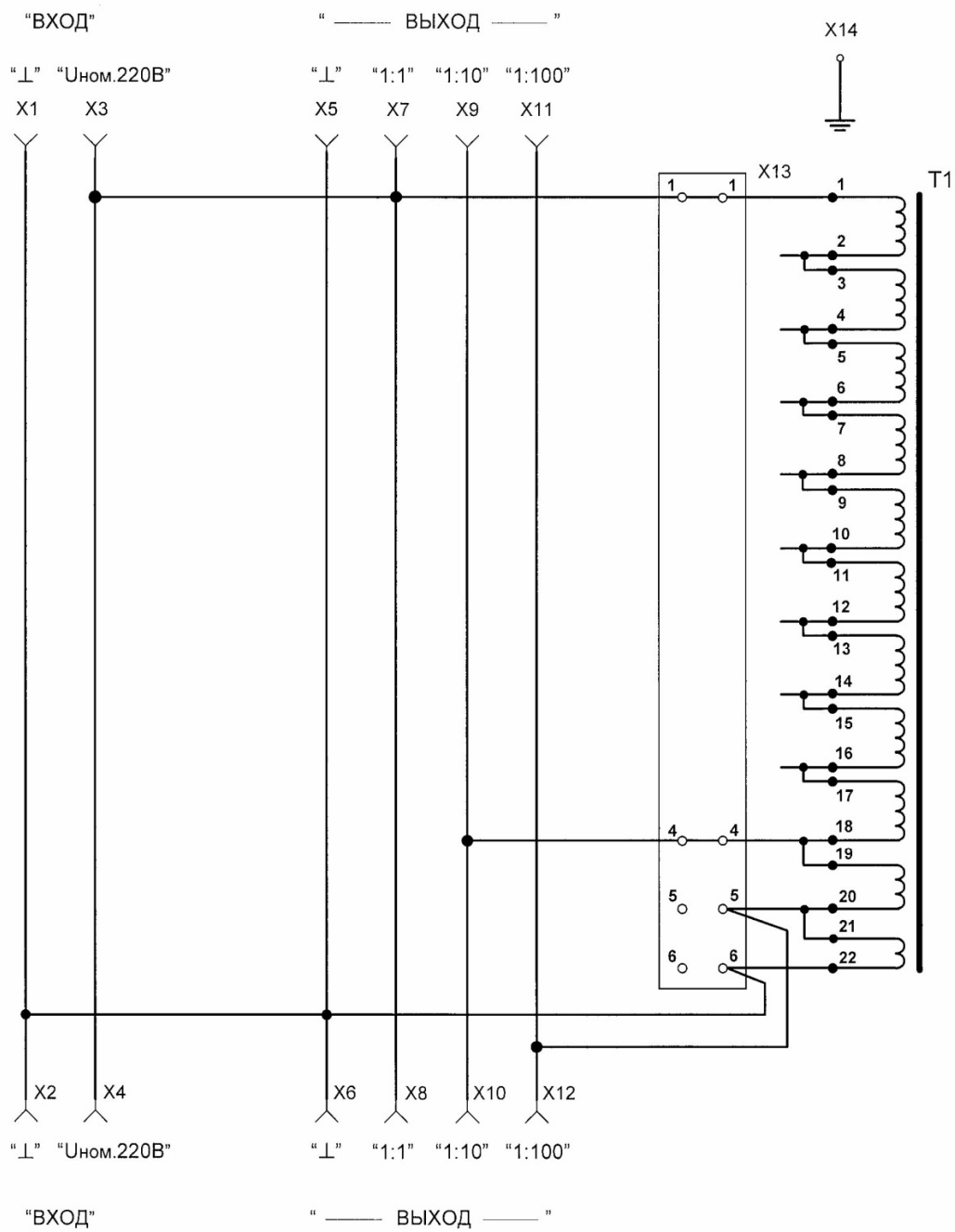
Рисунок 2.56 – Схема принципиальная ТП-1.0
