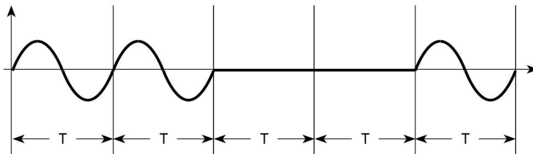
Рисунок 4.17 - Форма выходного сигнала в режиме «Субгармоники» (T — период сигнала)
