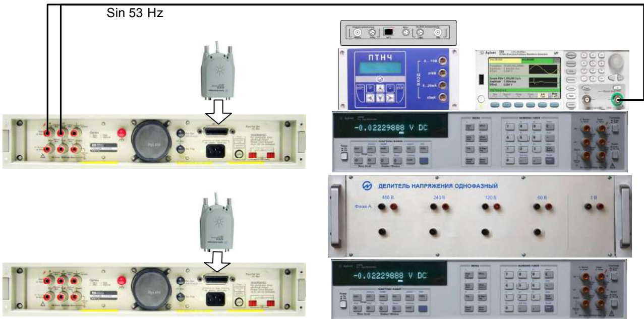
Рисунок А.7 - Схема цепи калибровки по частоте. HI – красный; LO - чёрный.
