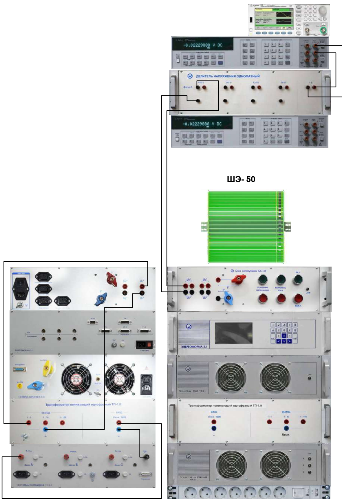
Рисунок А.4 - Схема измерительной цепи напряжения до 480 В
