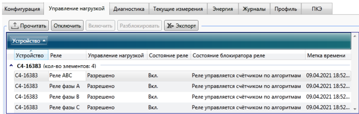
Рисунок 9.59 – Управление реле
