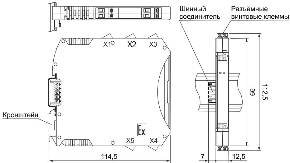
Рисунок 6.1 – Габаритные размеры барьера KA5011Ex-NN
