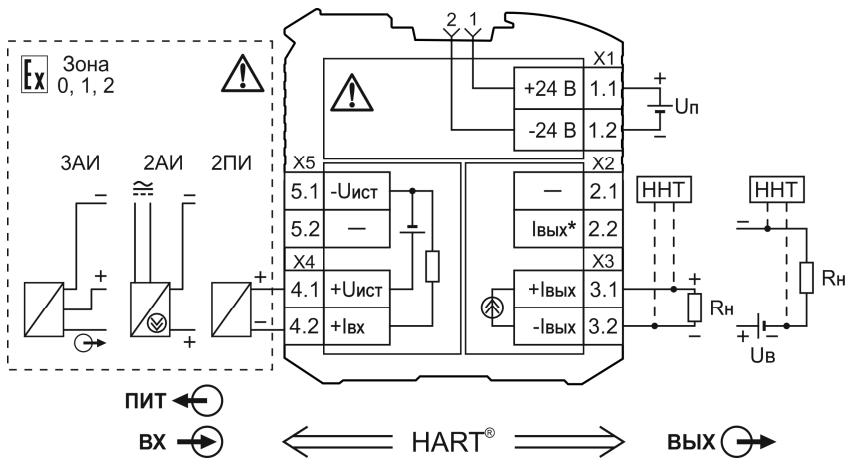
Рисунок 6.2 – Типовые схемы подключения барьеров KA5011Ex-NN
