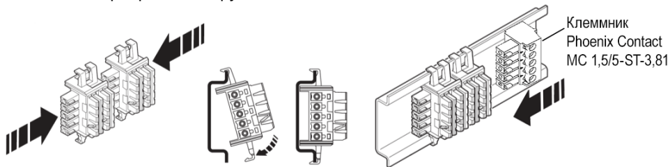
Рисунок 6.3 – Установка шинных соединителей на DIN- рейку
