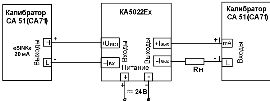
Рисунок 6.4.1А – Подключение барьеров мод. КА5022Ех для поверки преобразования входных унифицированных сигналов постоянного тока (входной пассивный сигнал) в диапазоне от 4 до 20 мА в выходной унифицированный сигнал постоянного тока от 4 до 20 мА
