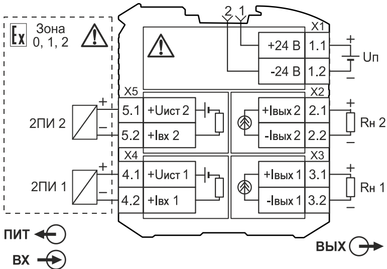
Рисунок 6.2 – Типовая схема подключения барьеров KA5022Ex-10
