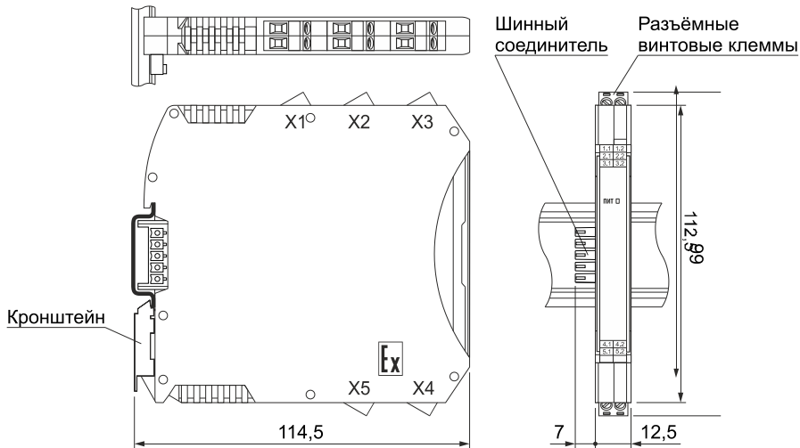
Рисунок 6.1 – Габаритные размеры барьера KA5022Ex-10
