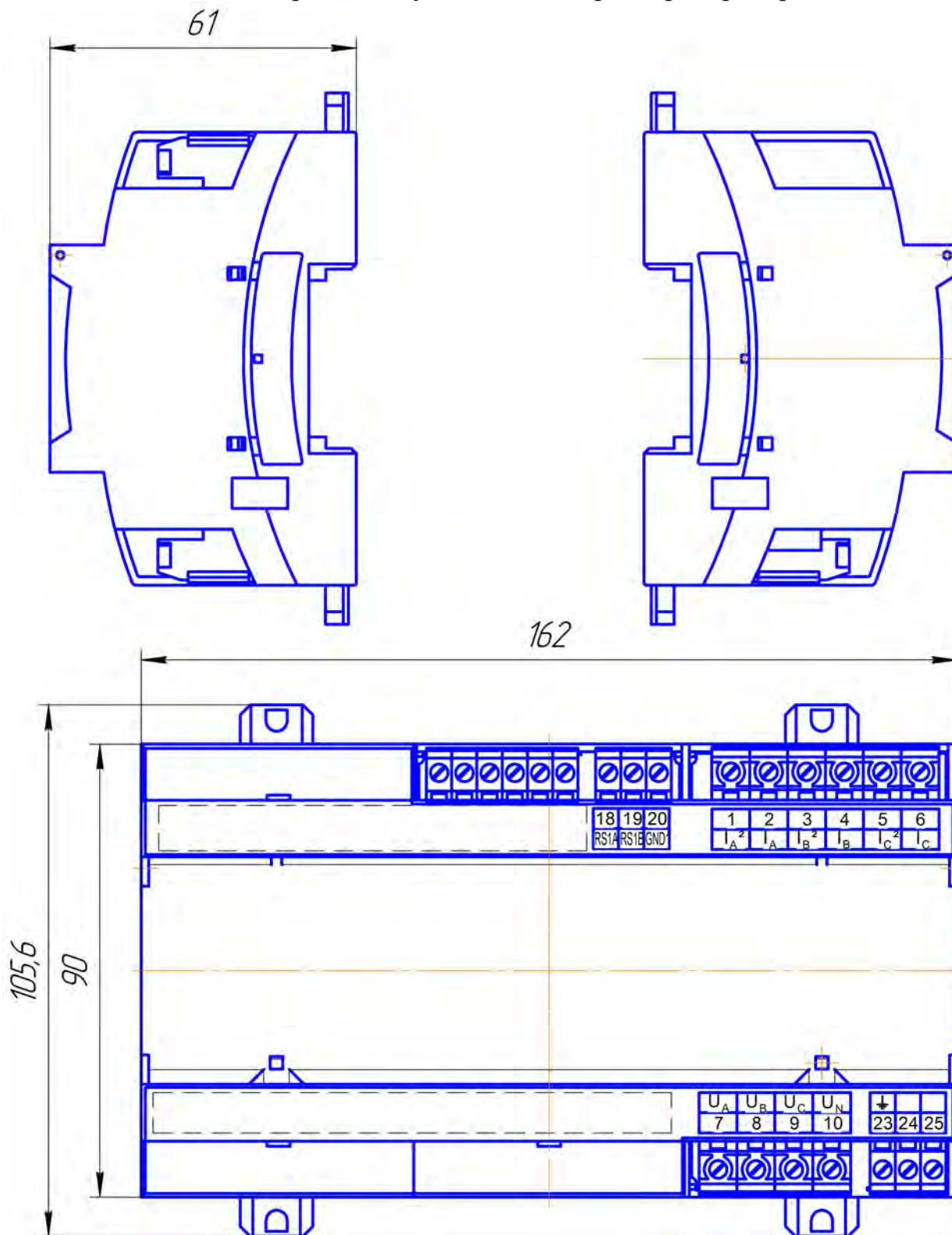
Рисунок А.1 – Общий вид, габаритные и установочные размеры (в мм) преобразователей серии Е
