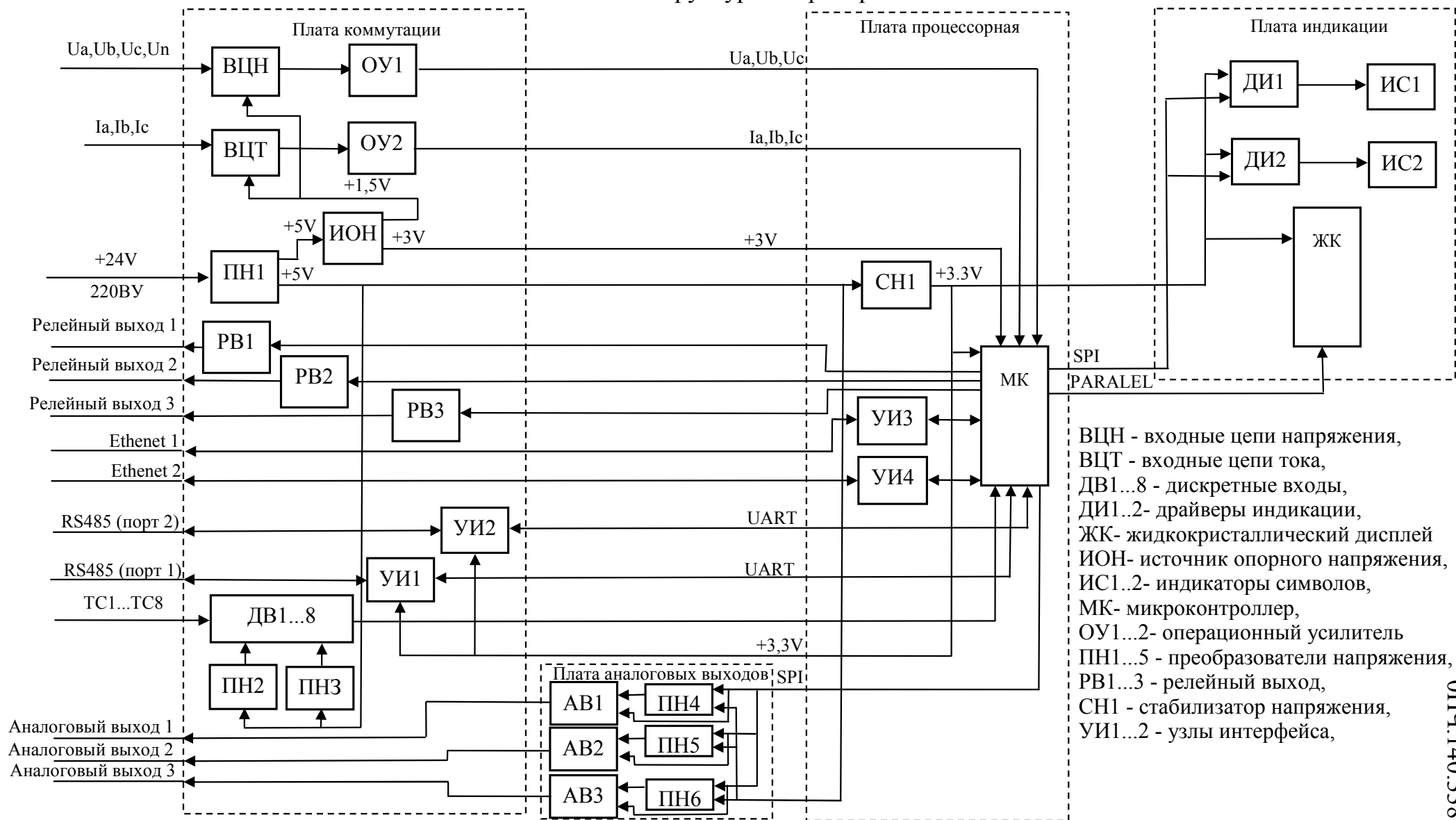
Рисунок В.1 – Схема структурная преобразователей
