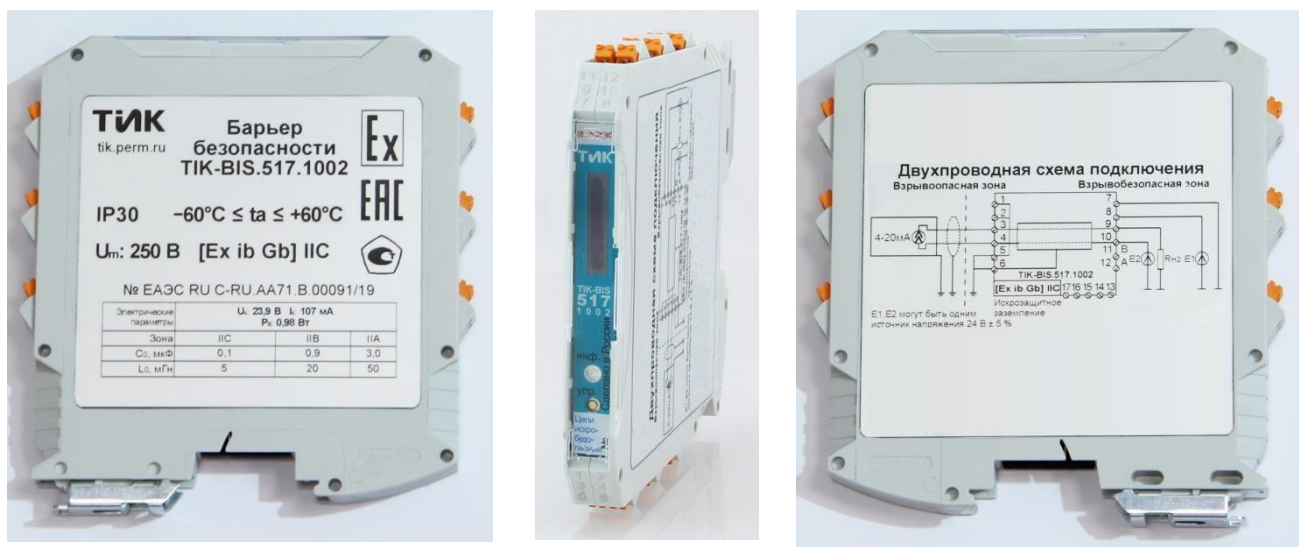
Рисунок 3 – Общий вид барьеров TIK-BIS.517.XXXX
