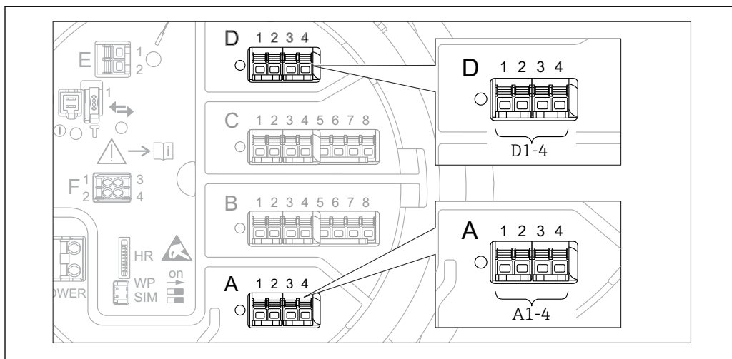
53 Обозначение модулей Modbus, V1 или WM550 (примеры). В зависимости от исполнения прибора эти модули могут находиться в гнезде B или C.
