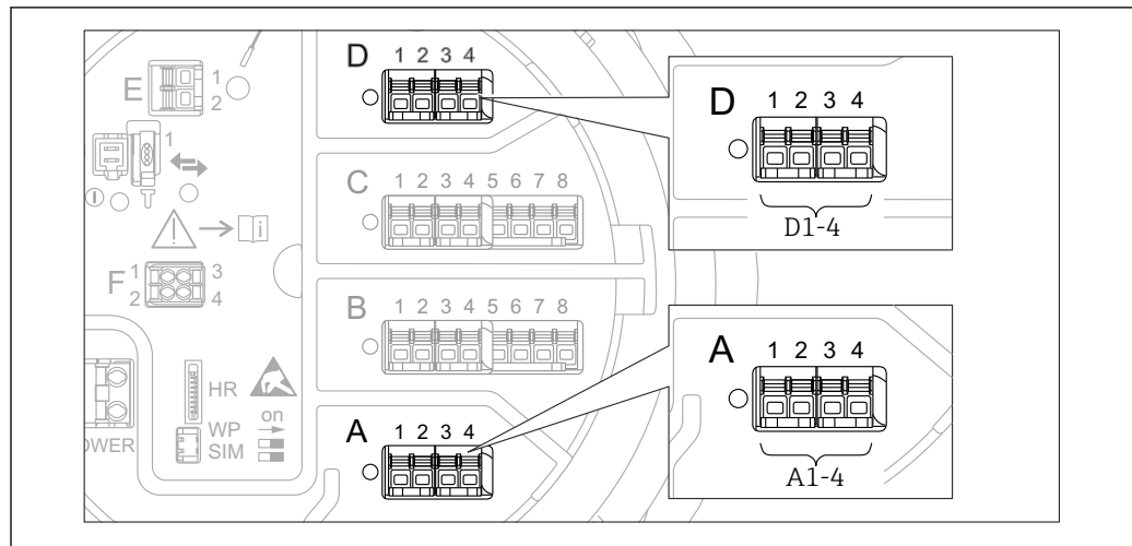
9 Обозначение модулей Modbus, V1 или WM550 (примеры). В зависимости от исполнения прибора эти модули могут находиться в гнезде В или С.
