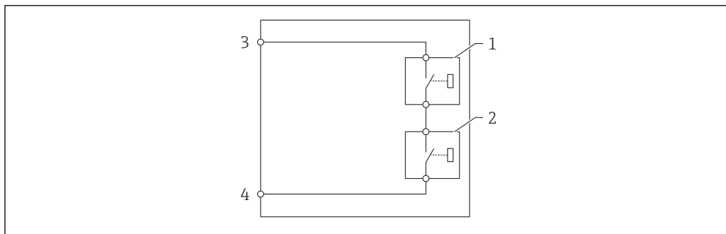
52 Два реле цифрового выхода
