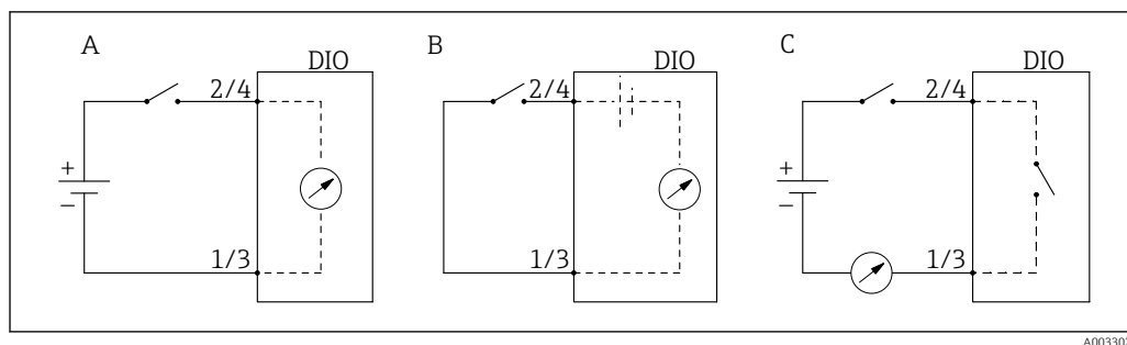
51 Режимы работы модуля цифрового ввода/вывода
