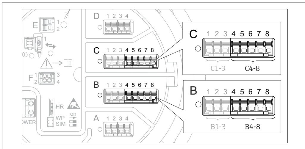
48 Контакты для подменю "Analog IP" (B4-8 или C4-8, соответственно)
