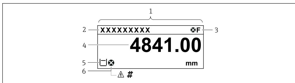
18 Типичный внешний вид основного экрана (индикация измеренного значения)
