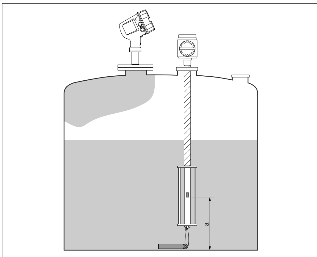
29 Позиция нижнего температурного элемента
