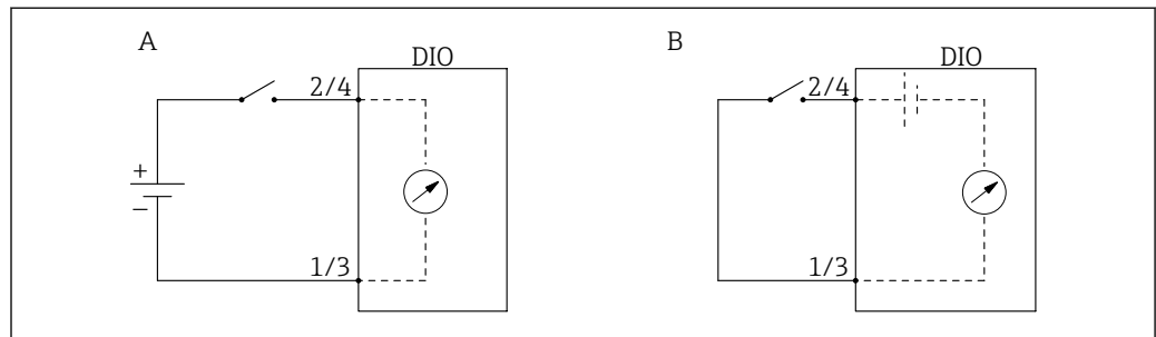
A «Режим работы» = «Вход пассивный» B «Режим работы» = «Ввод активен»
