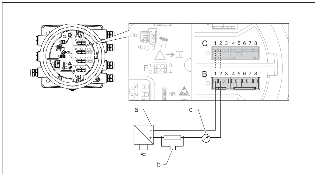
10 Использование модуля аналогового ввода/вывода в режиме пассивного выхода
