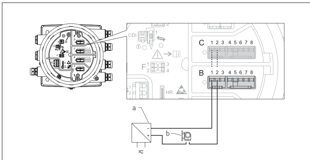
11 Использование модуля аналогового ввода/вывода в режиме пассивного входа
