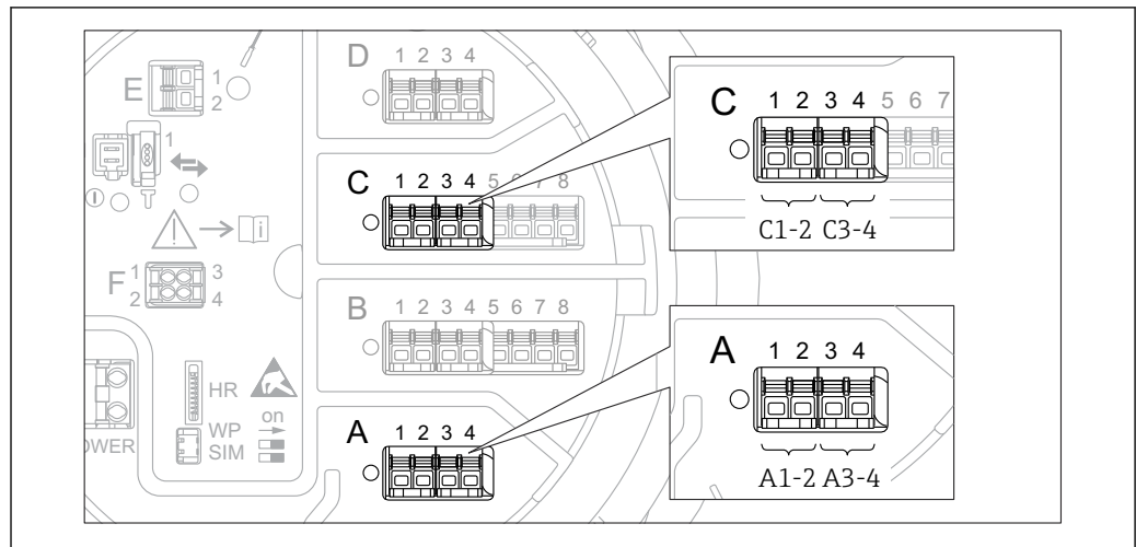
34 Возможное расположение цифровых модулей ввода/вывода (примеры); код заказа определяет номер и положение цифровых модулей ввода → 25.
