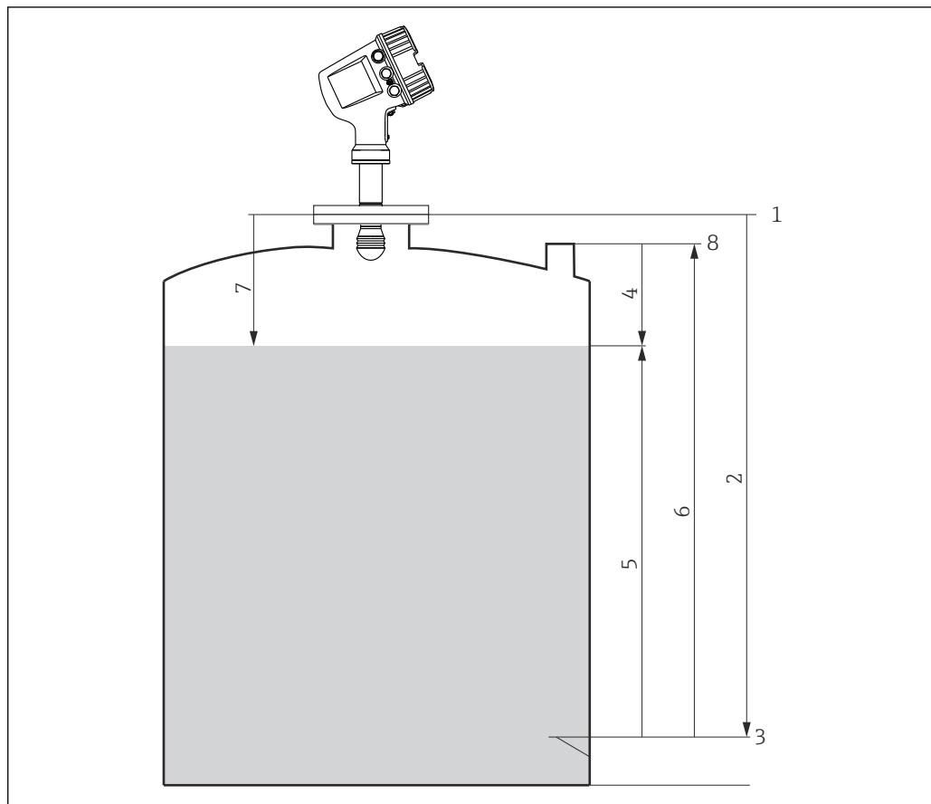
☑ 27 Термины, связанные с радарным измерением в резервуаре
