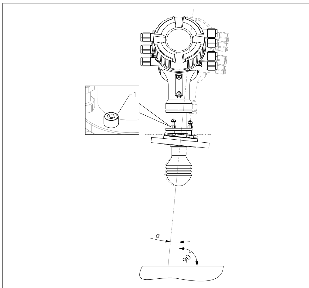
5 Приспособление для выравнивания на антенне 100 мм (4 дюйма)
