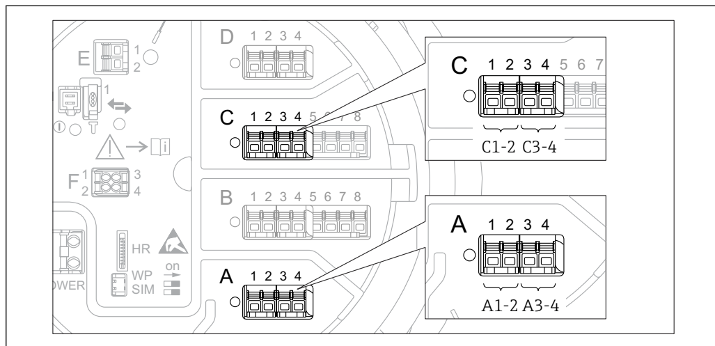
50 Обозначение цифровых входов и выходов (примеры)
