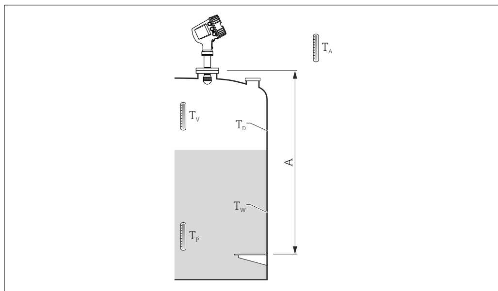
☐ 56 Параметры для вычисления значения CTSh
