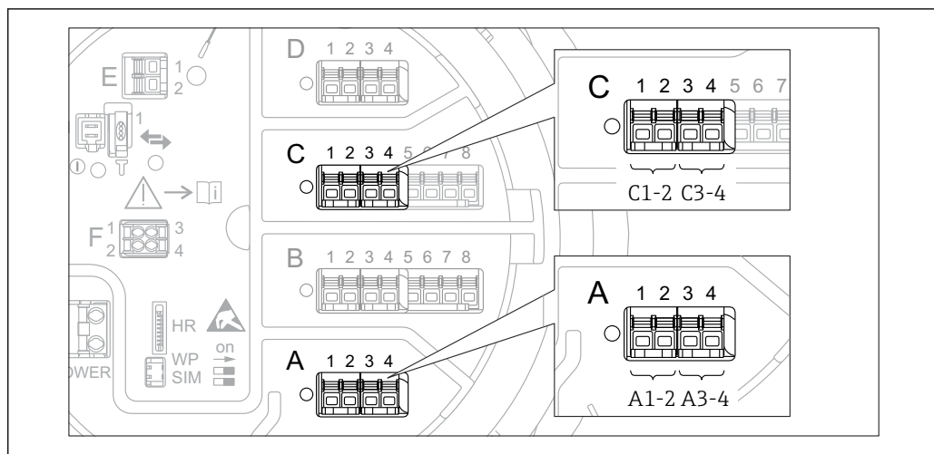
43 Возможное расположение цифровых модулей ввода/вывода (примеры); код заказа определяет номер и положение цифровых модулей ввода/вывода → 25.
