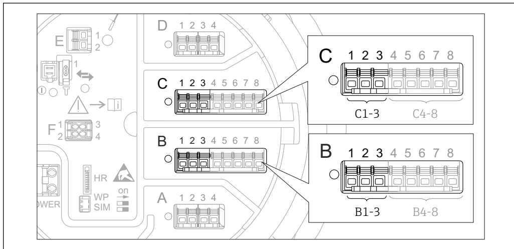
49 Контакты для подменю "Analog I/O" (B1-3 или C1-3, соответственно)
