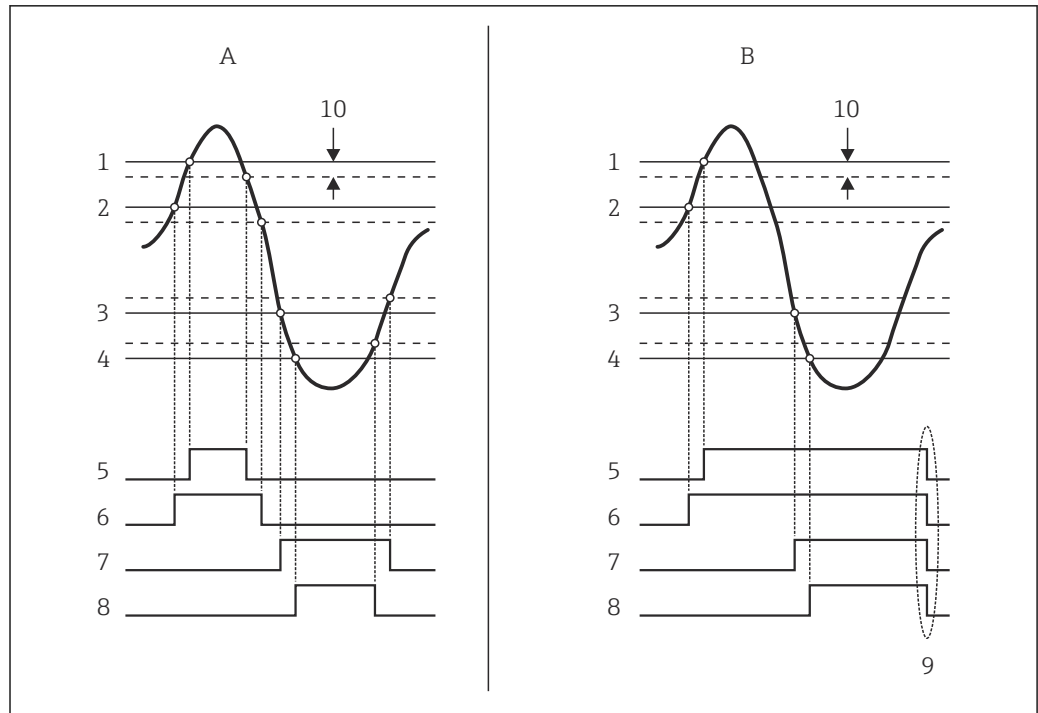
60 Принцип анализа предельных значений
