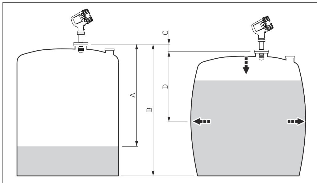
35 Коррекция гидростатической деформации резервуара (HyTD)
