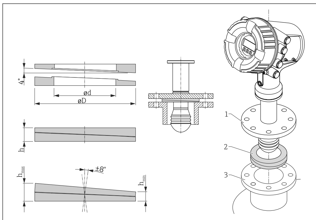
47 Регулируемое уплотнение используется для выравнивания прибора в пределах \pm 8 град
