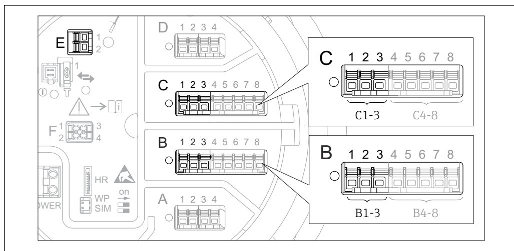
28 Доступные клеммы для цепей HART
