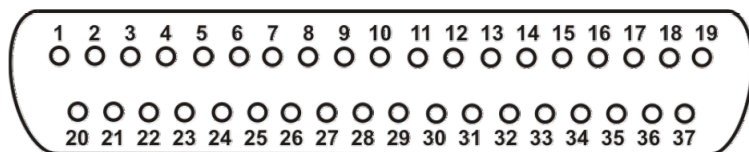
Разъём XRP1 (вид спереди)
