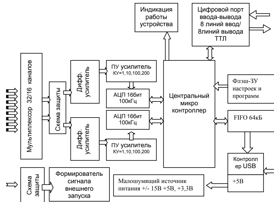
Рис. 10 Функциональная схема устройства прибора
