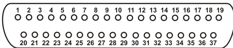
Разъём XP1 (вид спереди)
