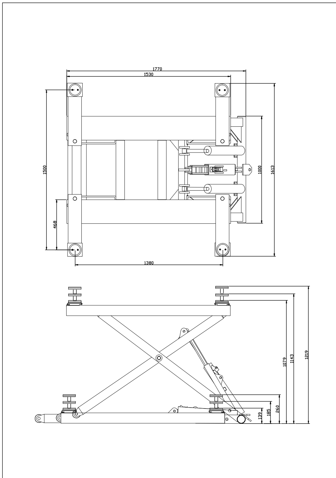
РИС. 2 - ЧЕРТЕЖ
