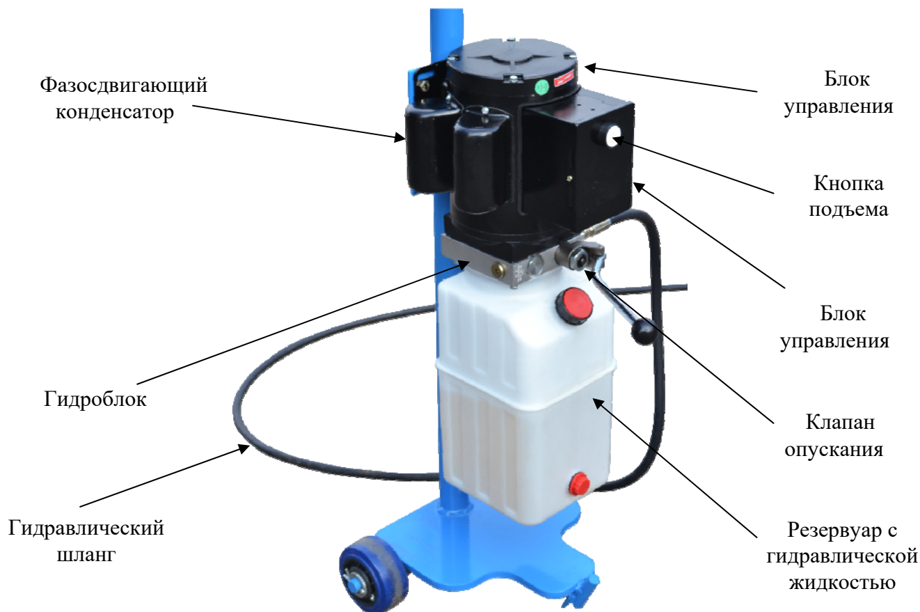
РИС. 3 - ГИДРАВЛИЧЕСКИЙ АГРЕГАТ
