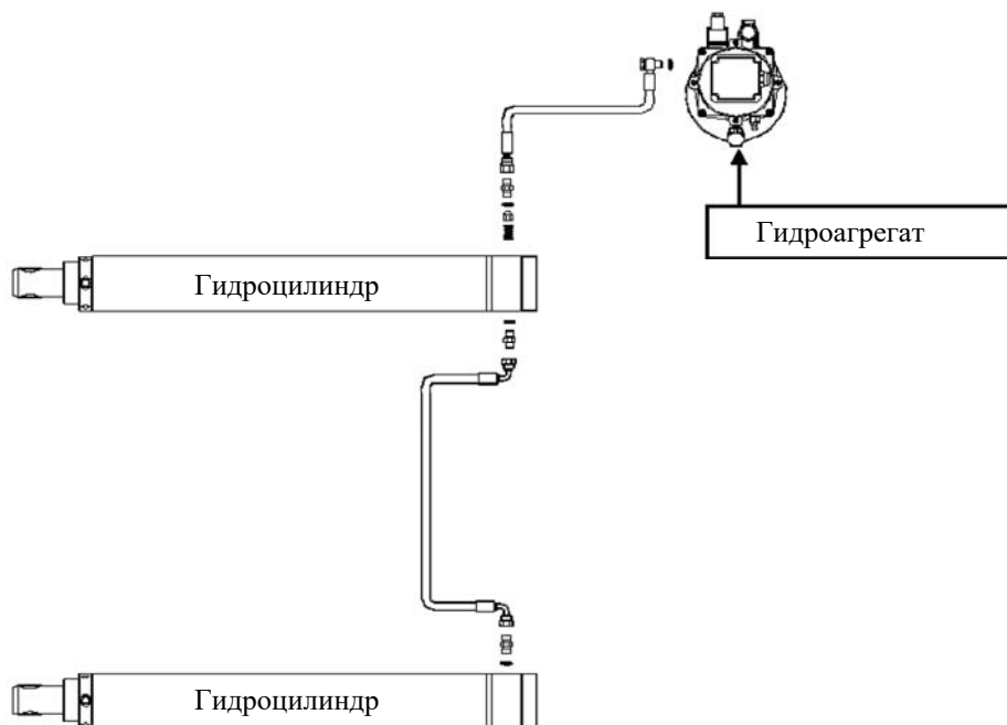
РИС. 5 – ГИДРАВЛИЧЕСКАЯ СИСТЕМА
