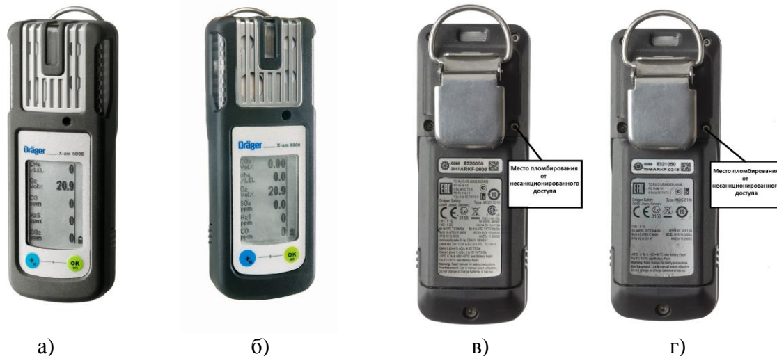
Рисунок 1 – Общий вид газоанализаторов портативных: а) Dräger X-am 5000 тип MQG 0010; б) Dräger X-am 5600 тип MQG 0100; схема пломбирования: в) Dräger X-am 5000 тип MQG 0010; г) Dräger X-am 5600 тип MQG 0100
