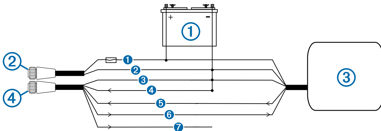
Устройство с одним выходом, совместимое с NMEA 0183
