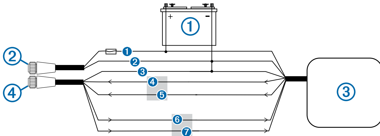
Устройство, совместимое со стандартом NMEA 0183, подключенное для односторонней передачи данных
