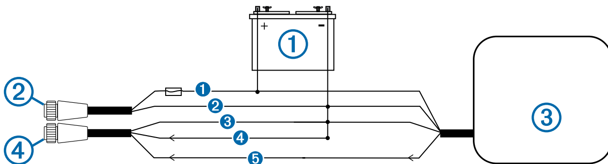
Устройство, совместимое со стандартом NMEA 0183, с одним подключенным проводом для передачи данных
