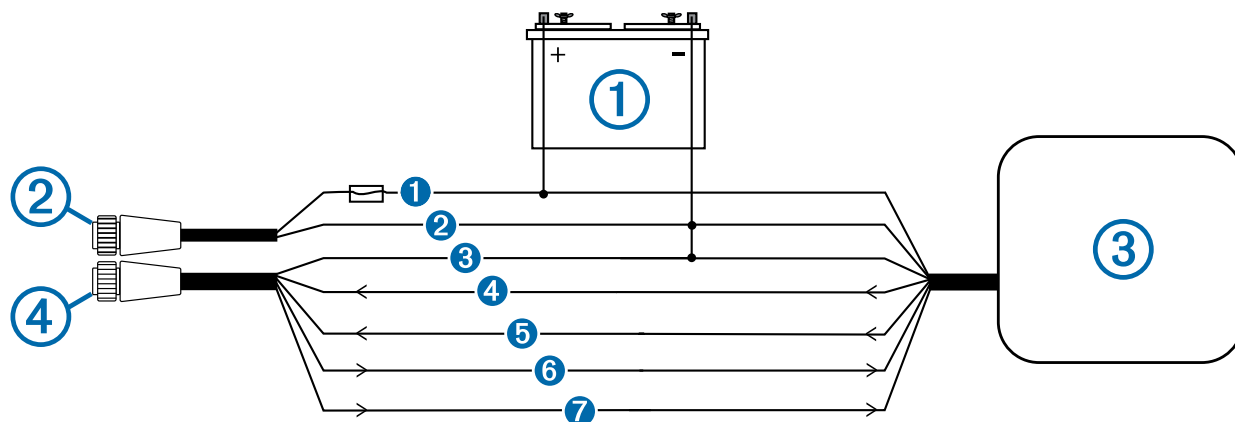
Устройство, совместимое со стандартом NMEA 0183, подключенное для двусторонней передачи данных
