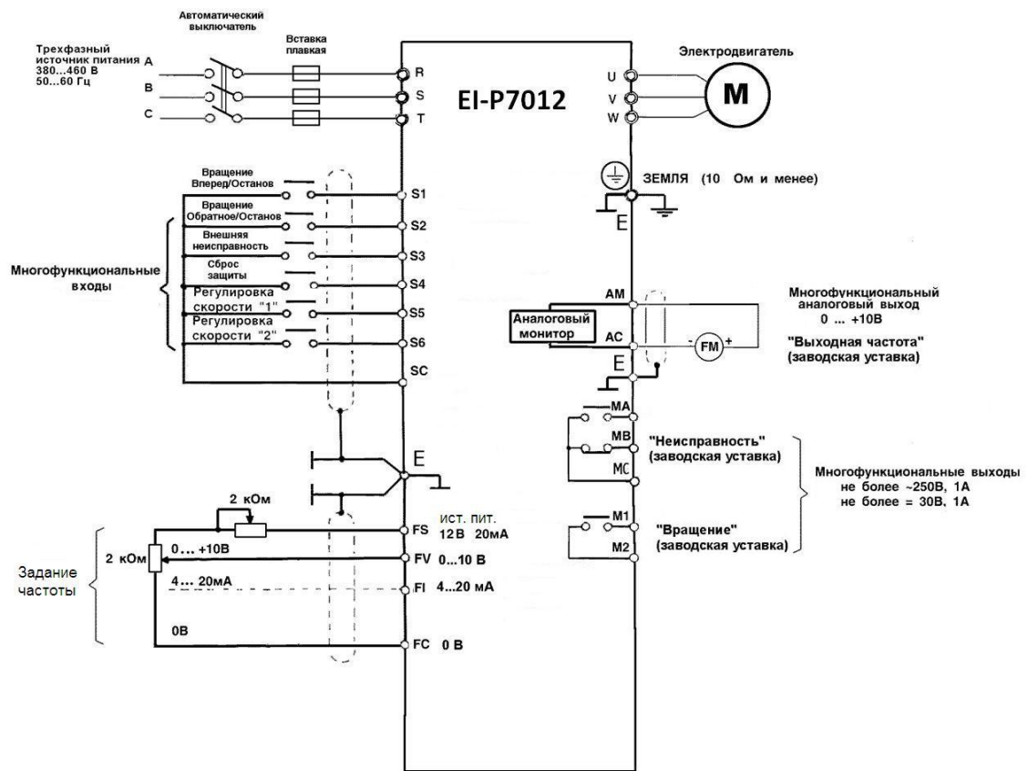
Рис. 9. Схема подсоединения.
