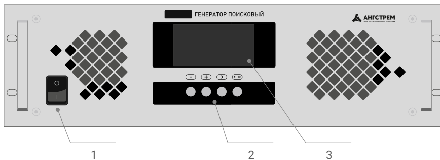
Рисунок 1 - Передняя панель генератора
