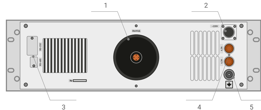
Рисунок 2 - Задняя панель генератора
