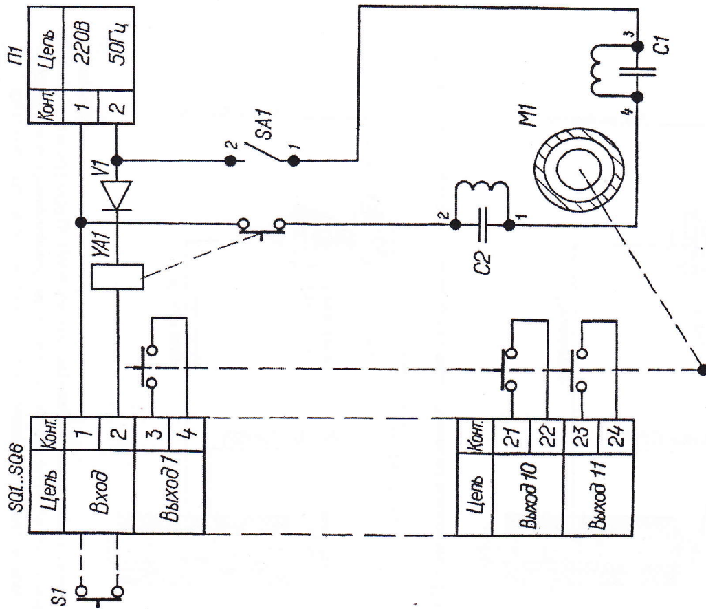
П1 – панель питания; SA1 – тумблер ТВ2-1; S1 - выключатель; YA1 – электромагнит; SQ1 – SQ6 – контактная группа; M1 – электродвигатель СД-54 (I/137); C1 – конденсатор МБГЧ-1-2А-250-0,5±10%; C2 – конденсатор МБГЧ-1-2А-250-2,0±10%; V1 – диод Д226Б.
