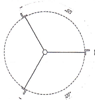
Рисунок 1 – Схема размещения растяжек в плане
