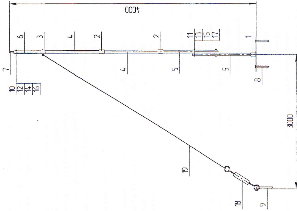
1 – основание; 2 – втулка; 3 – втулка; 4 – стойка; 5 – стойка; 5 – стойка; 6 – стойка; 7 – штырь; 8 – штырь; 9 – штырь; 10 – болт; 11 – болт; 12 – гайка; 13 – гайка; 14 – шайба; 15 – шайба; 16 – шайба; 17 – шайба; 18 – талреп; 19 – растяжка
