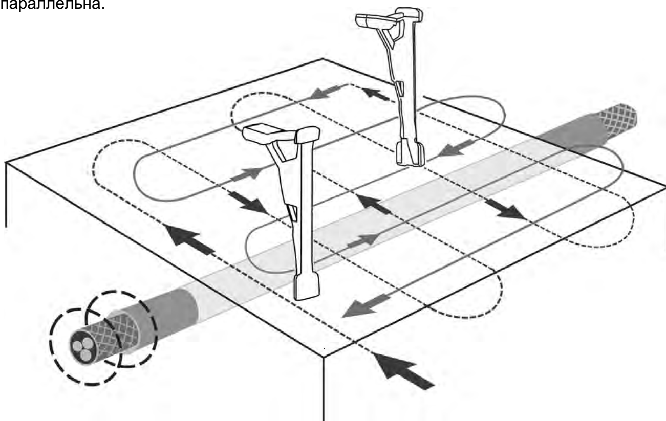
Рисунок 4.4.1 – Обследование участков местности без генератора
