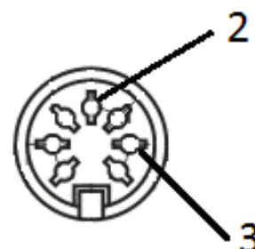
Рисунок 13.5.4 – Нумерация контактов гнезда «ДАТЧИК»
