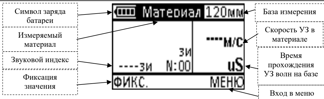
Рисунок 2.7 – Режим измерения звукового индекса
