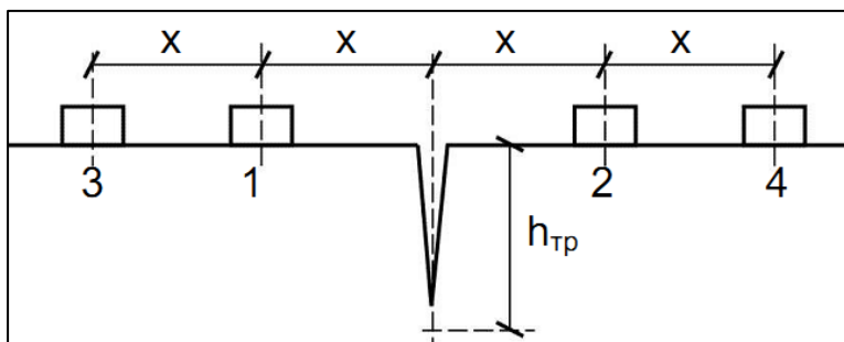
Рисунок 2.14 – Схема установления преобразователей для британской методики
