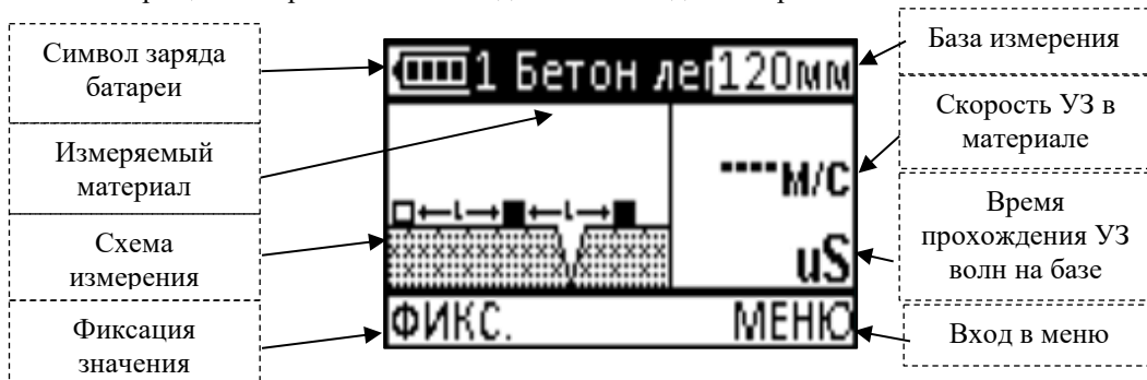
Рисунок 2.8 – Режим определения глубины трещины по российской методике
