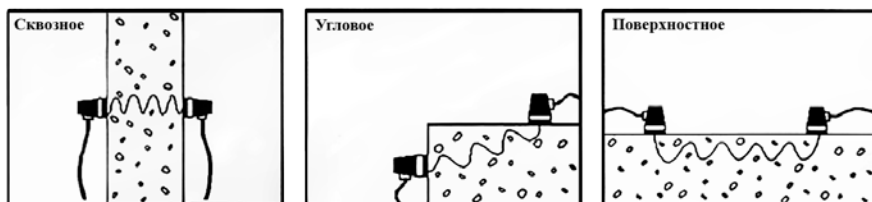
Рисунок 1.3 – Методы прозвучивания со смазкой
