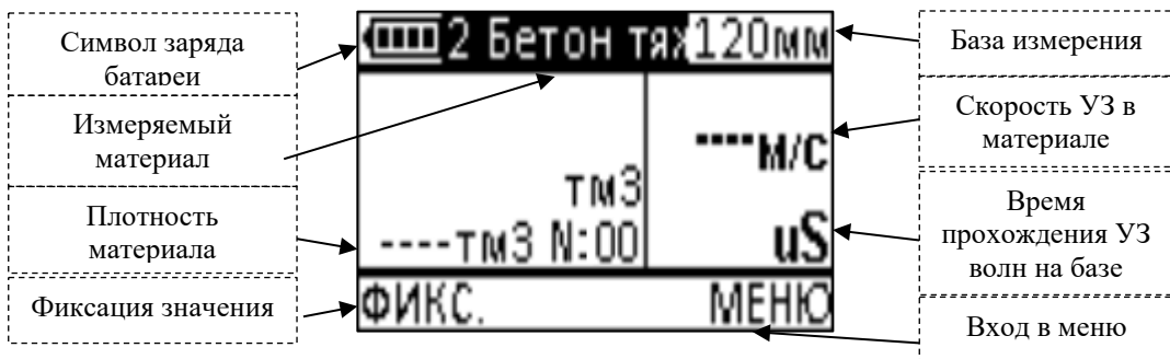
Рисунок 2.5 – Режим измерения плотности
