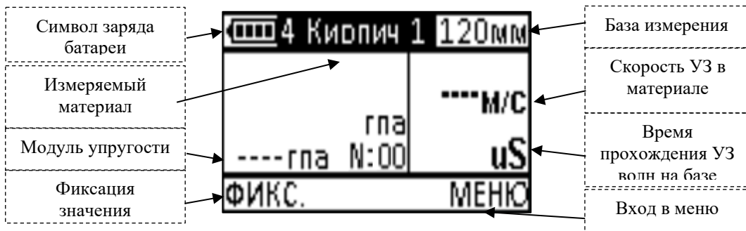
Рисунок 2.6 – Режим измерения модуля упругости
