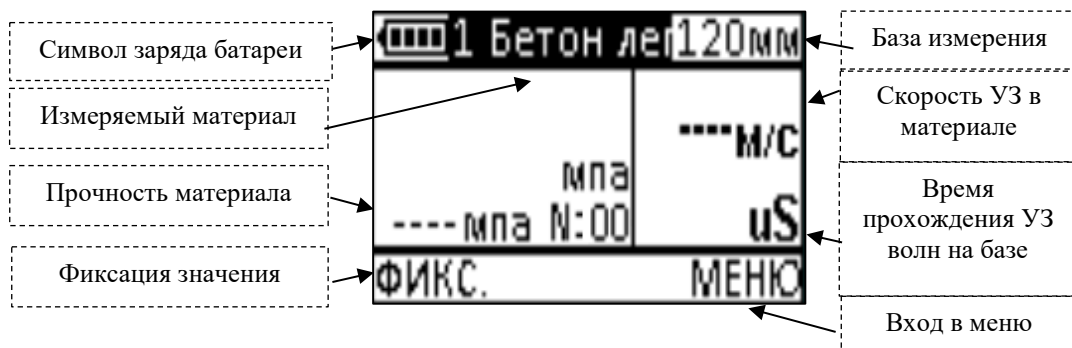
Рисунок 2.4 – Режим измерения прочности
