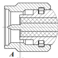
SMA, вилка
