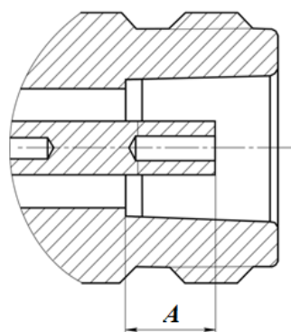
N, розетка
