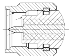
SMA, вилка
