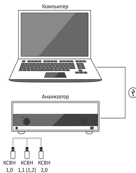
Рисунок А.13 – Схема измерений
