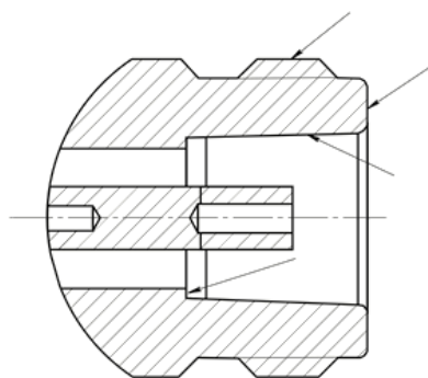
N, розетка
