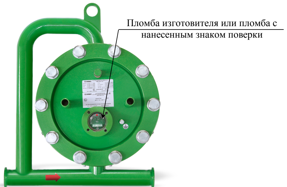
Рисунок 1 – Схема пломбировки счетчиков моноблочного и раздельного исполнения
