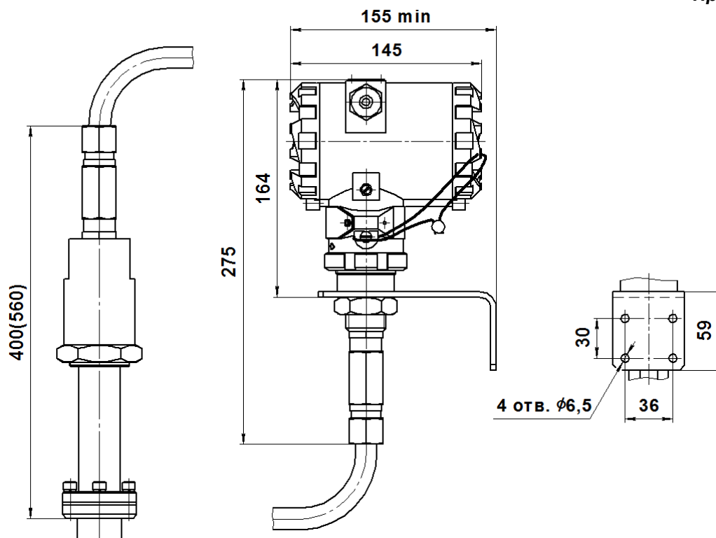
Рисунок В.10 - Размеры преобразователей дистанционного исполнения. Остальные размеры см. Рис.В.1 ...В.10
