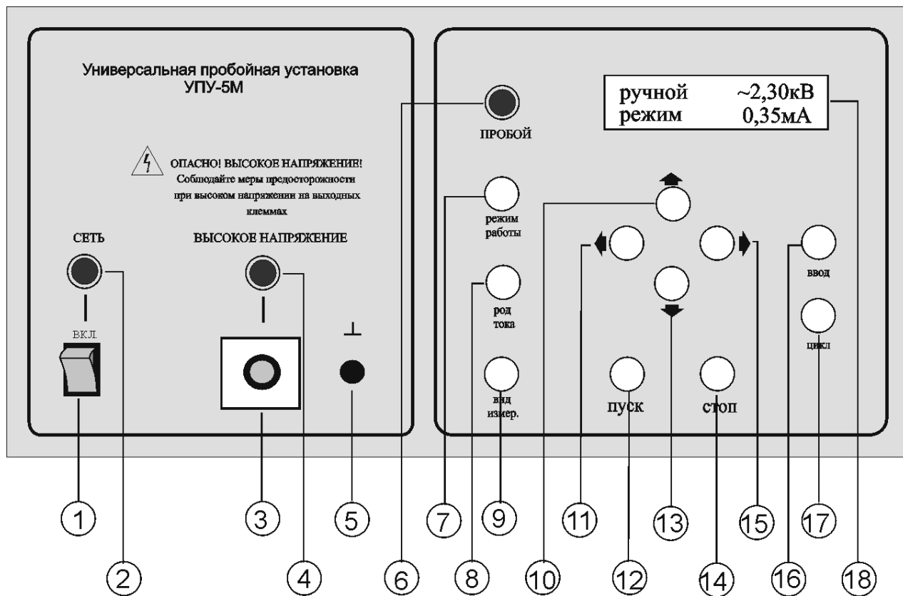
рис. 1 Передняя панель
