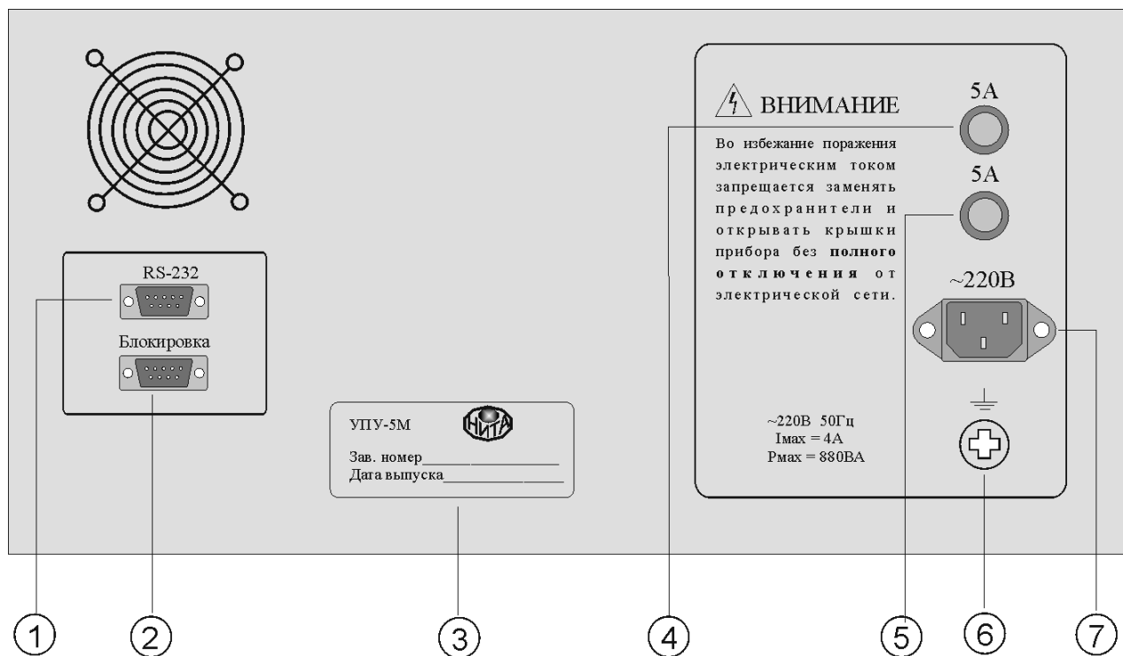
рис. 2 Задняя панель
