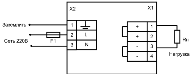
Рисунок 2 – Схема подключения блока питания
