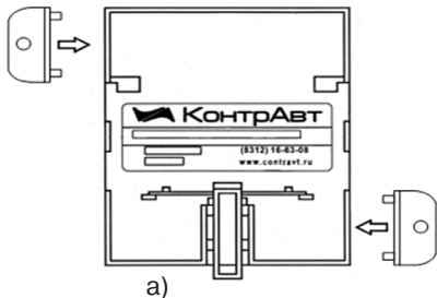
Рисунок 4 – Способы установки блока питания при монтаже
