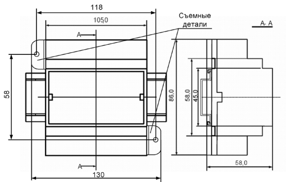
Рисунок 3 – Габаритные и присоединительные размеры блока питания PSM-72-24
